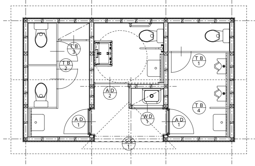
建具キープラン SC.1/50
