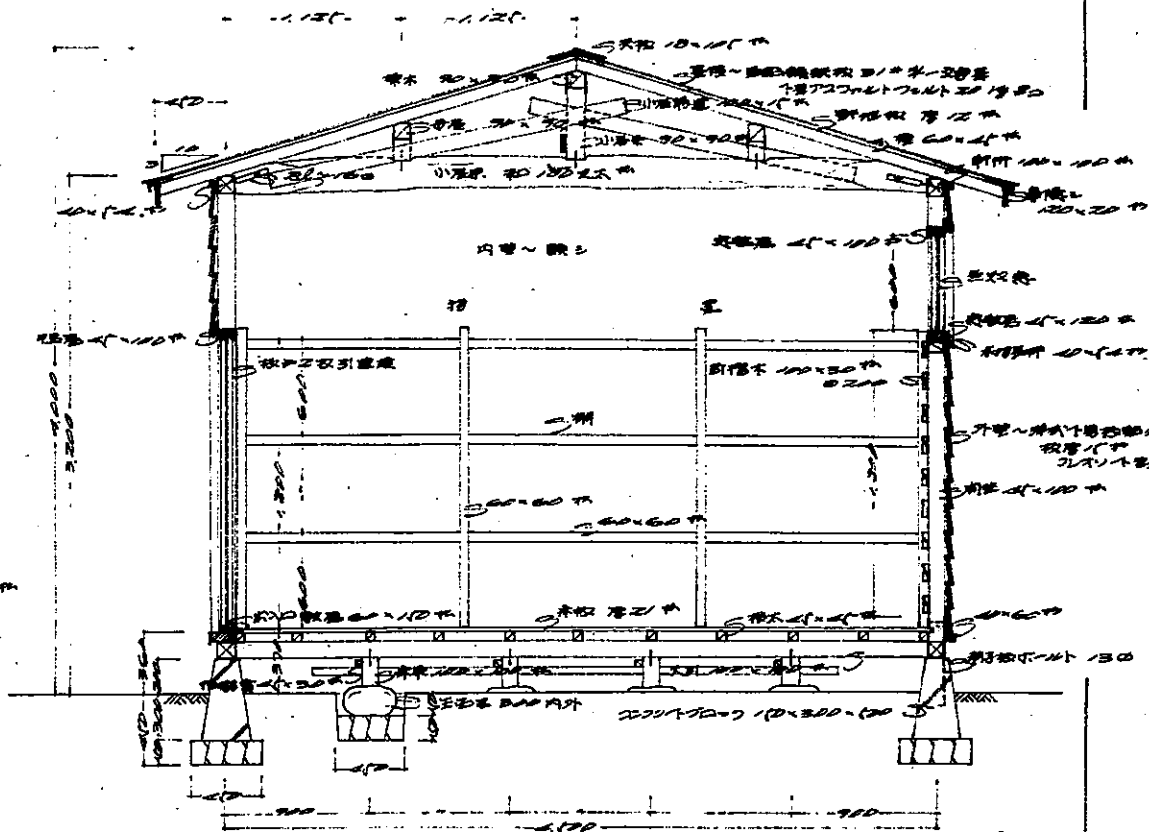
切斷圖 1/30
