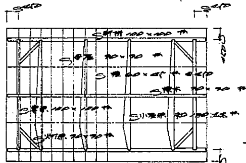
木次圖 1/100
