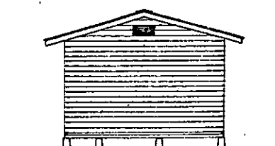
南北側立面圖 1/100
