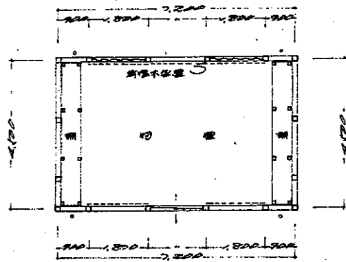
平面圖 1/100 ○~ 附屬法室 (柱-1/2)
