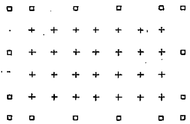
基礎柱圖 1/100
