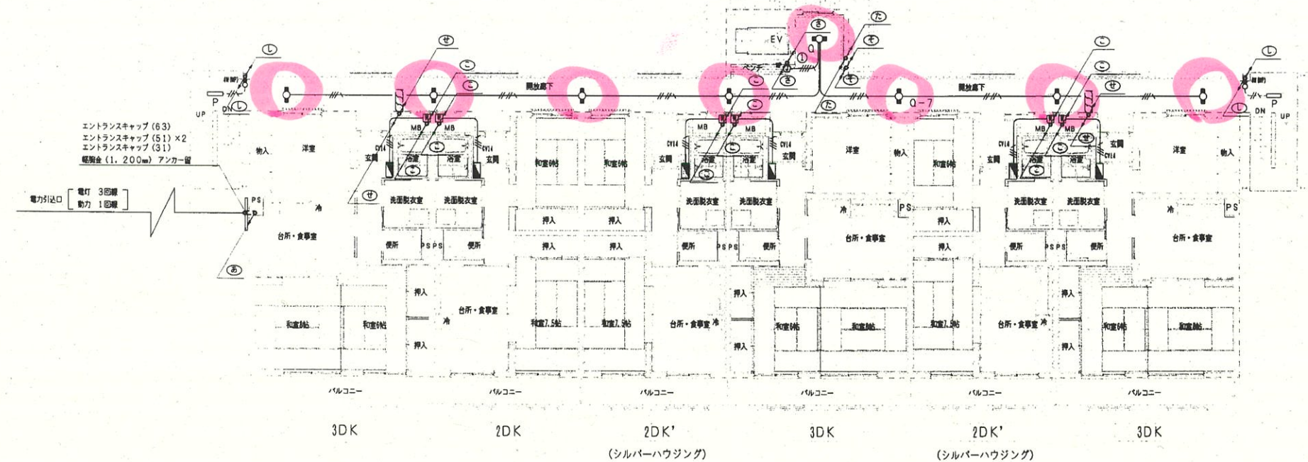
2階配線図 1 : 100
