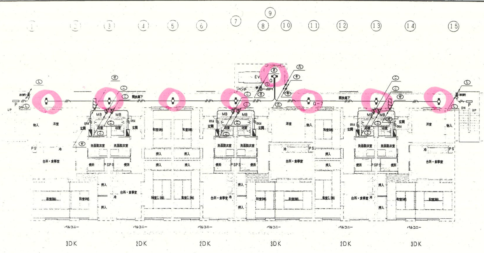
3階配線図 1 : 100
