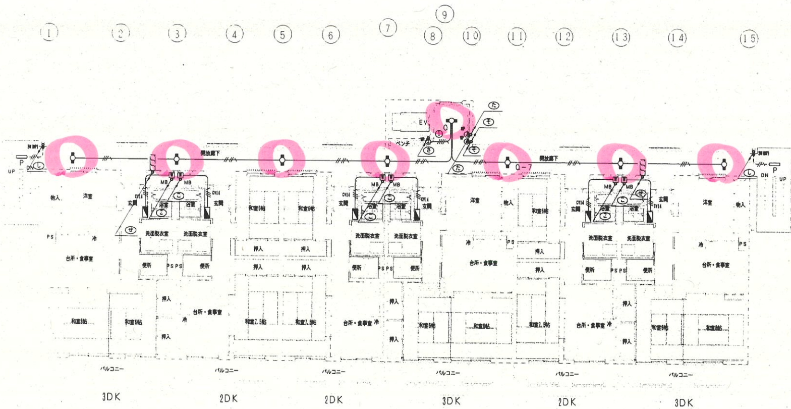
4階配線図 1 : 100
