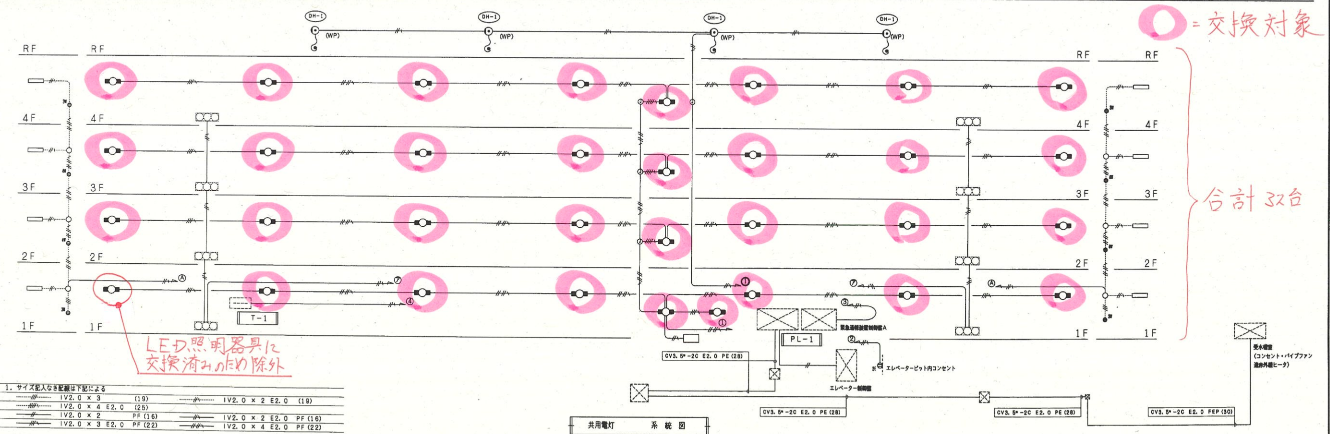
幹線・動力設備 系統図
