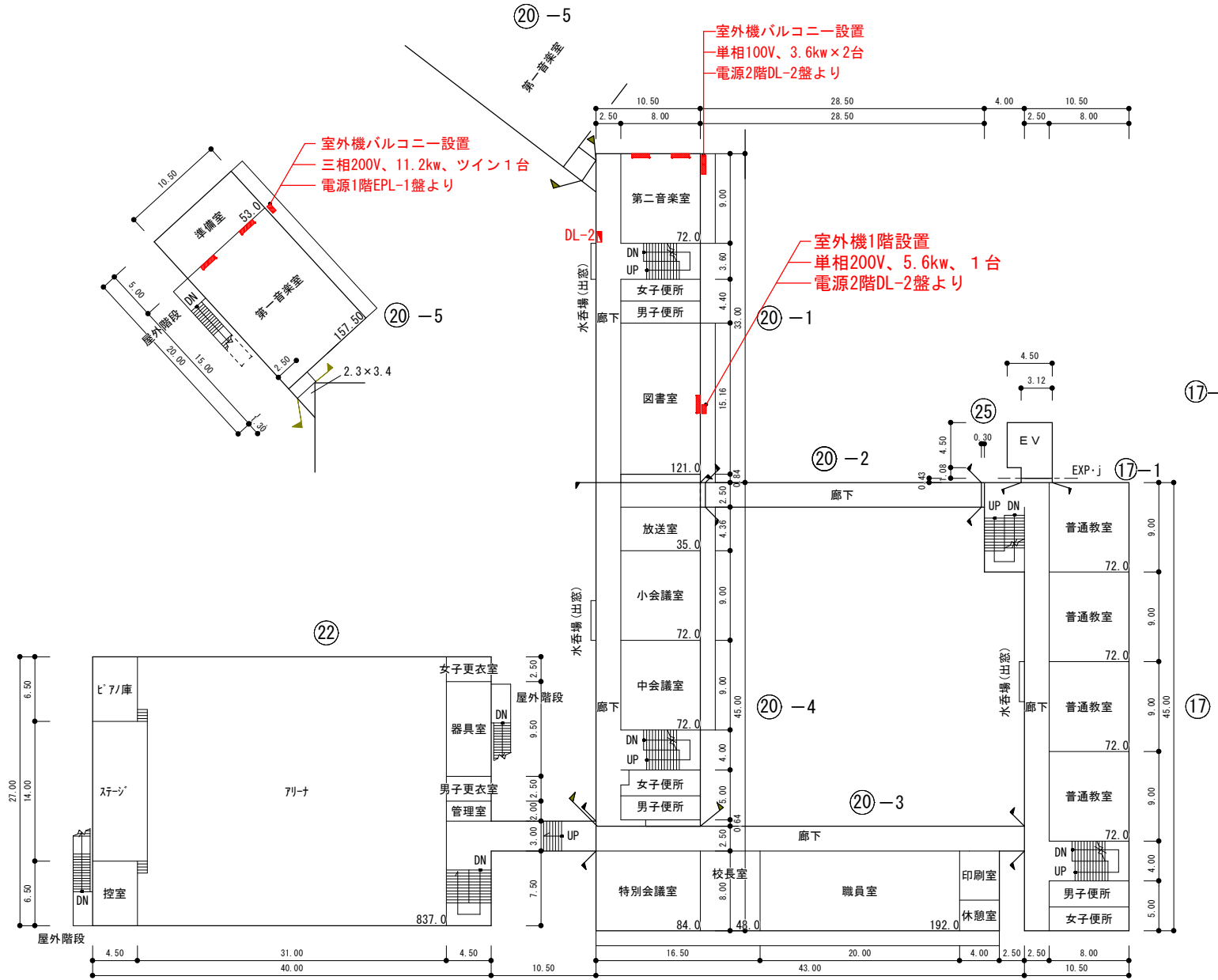
2階平面図
