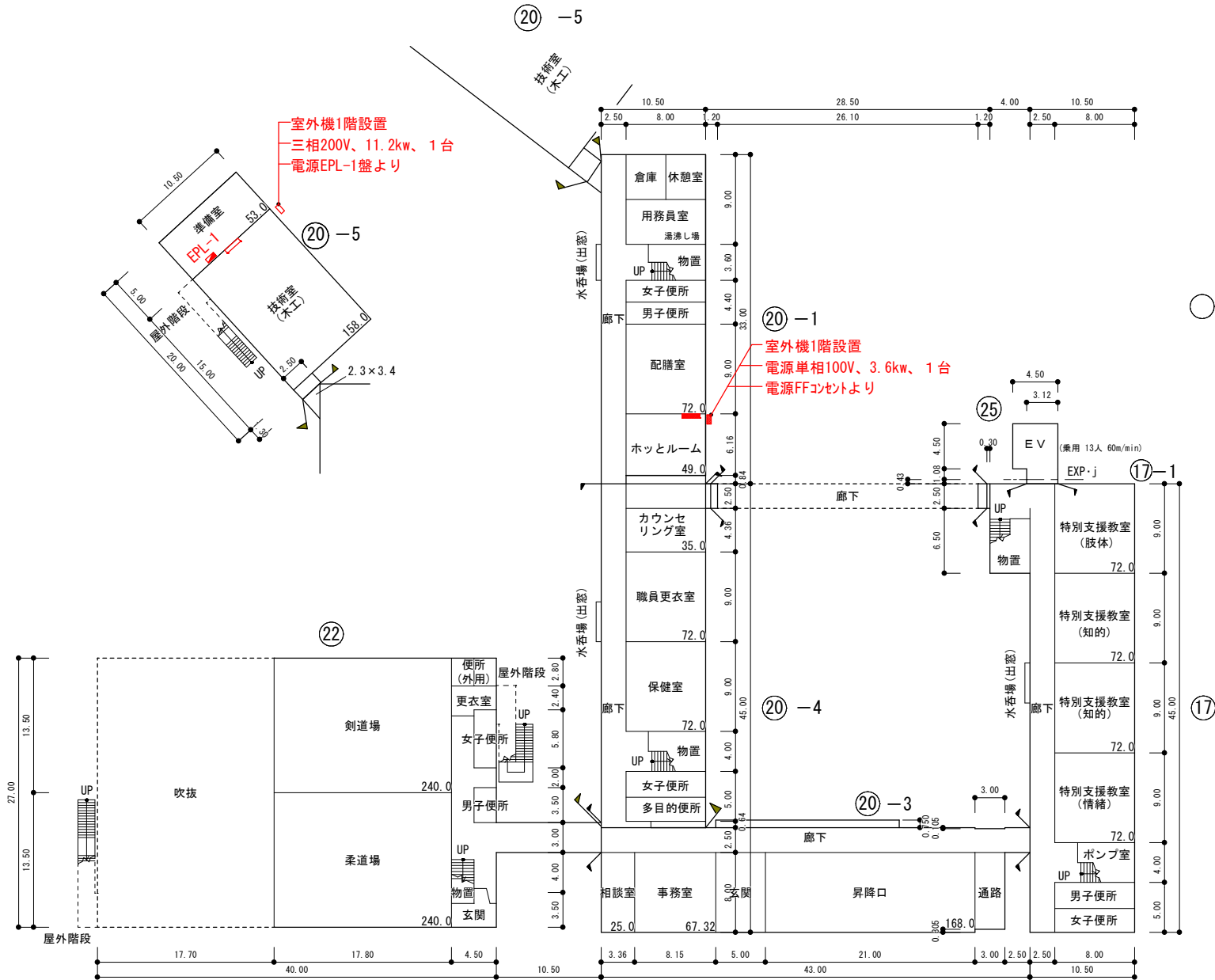
1 階 平 面 図
