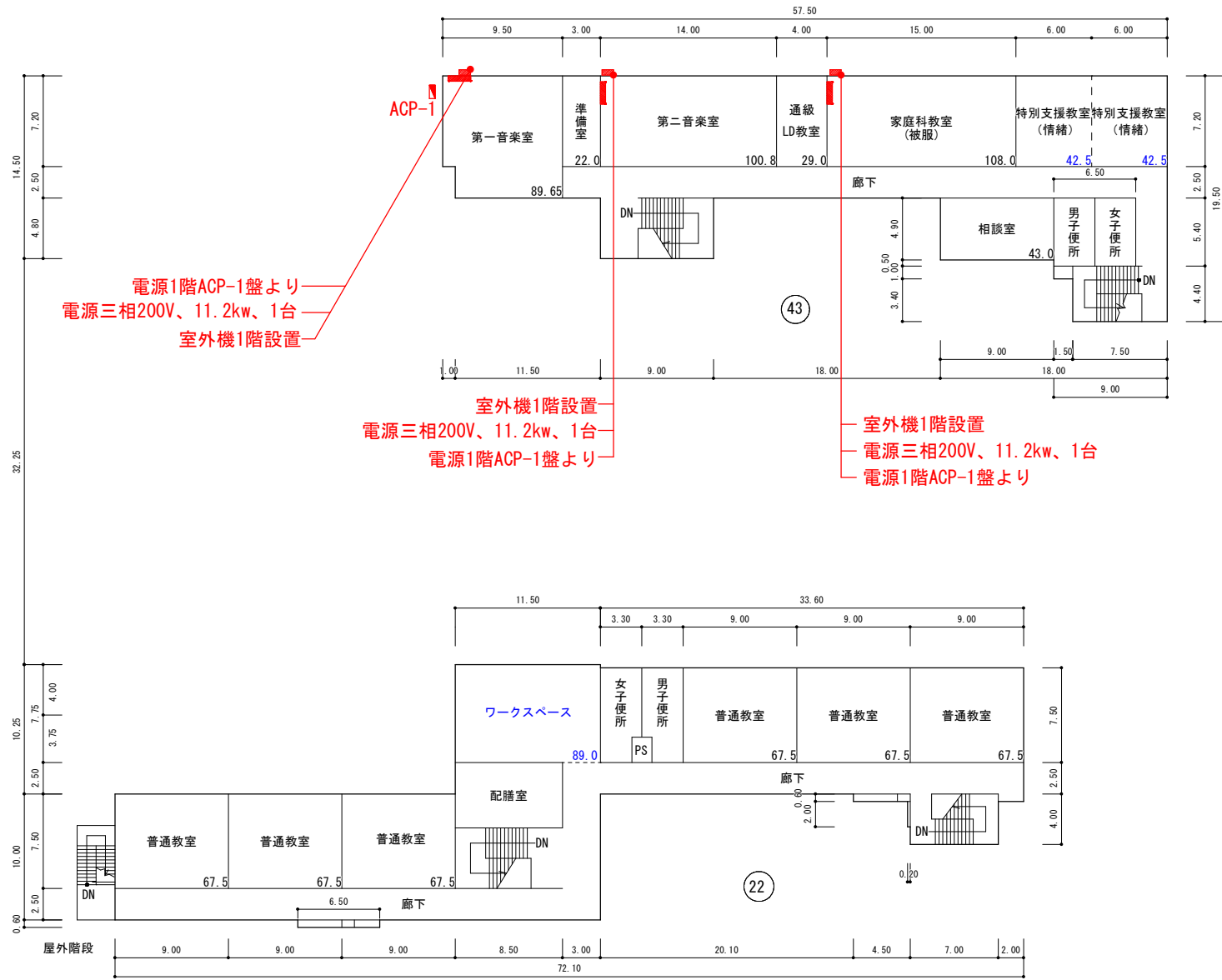
3 階 平 面 図
