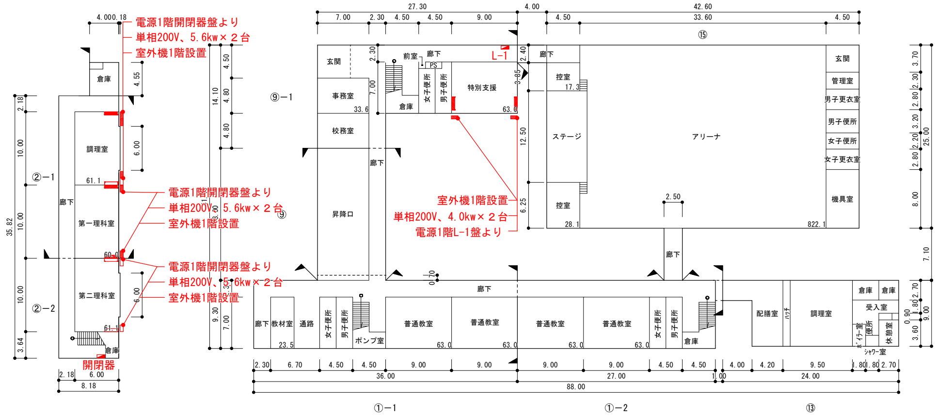
1 階 平 面 図
