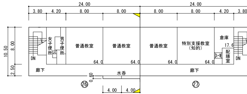
4 階 平 面 図
