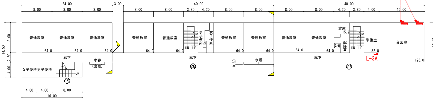
3 階 平 面 図
