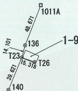
基準点網図 S=1/2500
