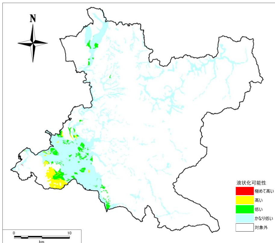
北上低地西縁断層帯型地震(内陸活断層による地震)液状化危険度分布図
