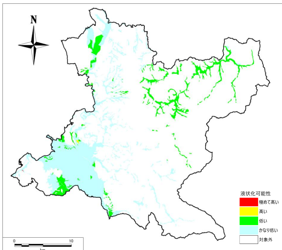
東北地方太平洋沖型地震(海溝型地震)液状化危険度分布図
