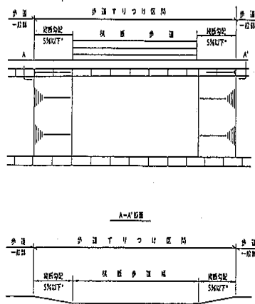
参考図 IV-4 歩道の車道とのすり付け構造 (横断歩道箇所—交差点に横断歩道がある場合)
