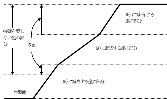
図 2-6 連続した崖
