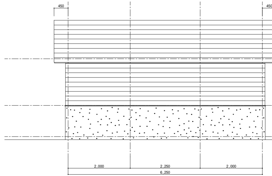
東側立面図 SC/1:50
