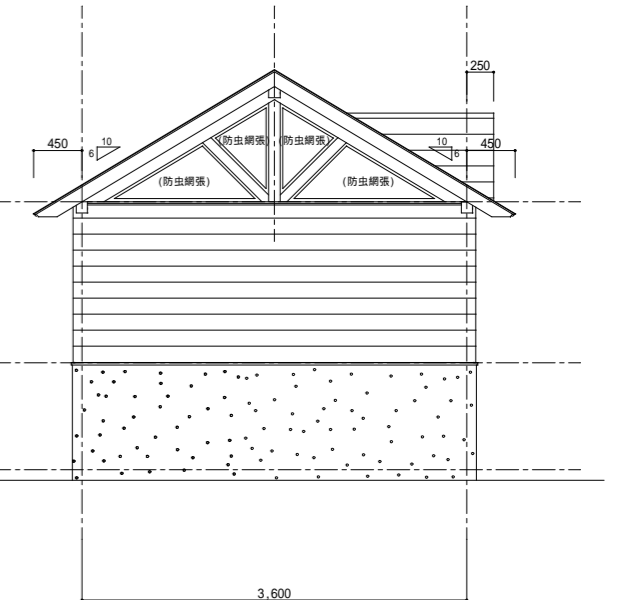
北側立面図 SC/1:50
