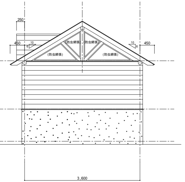
南側立面図 SC/1:50
