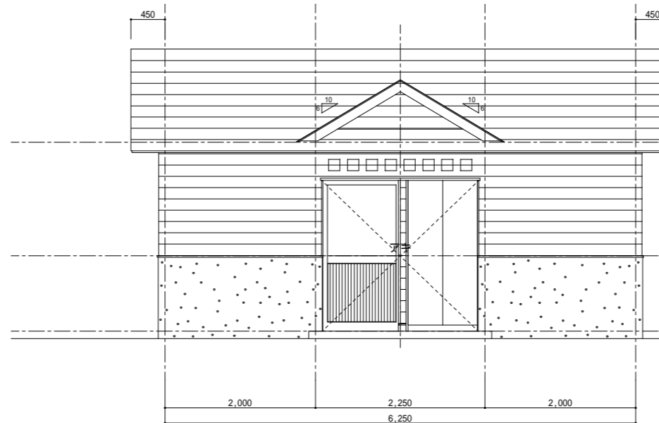
西側立面図 SC/1:50
