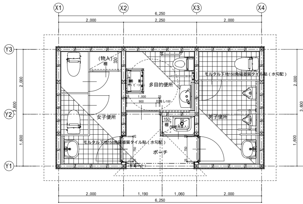
平面図 SC/1:50
