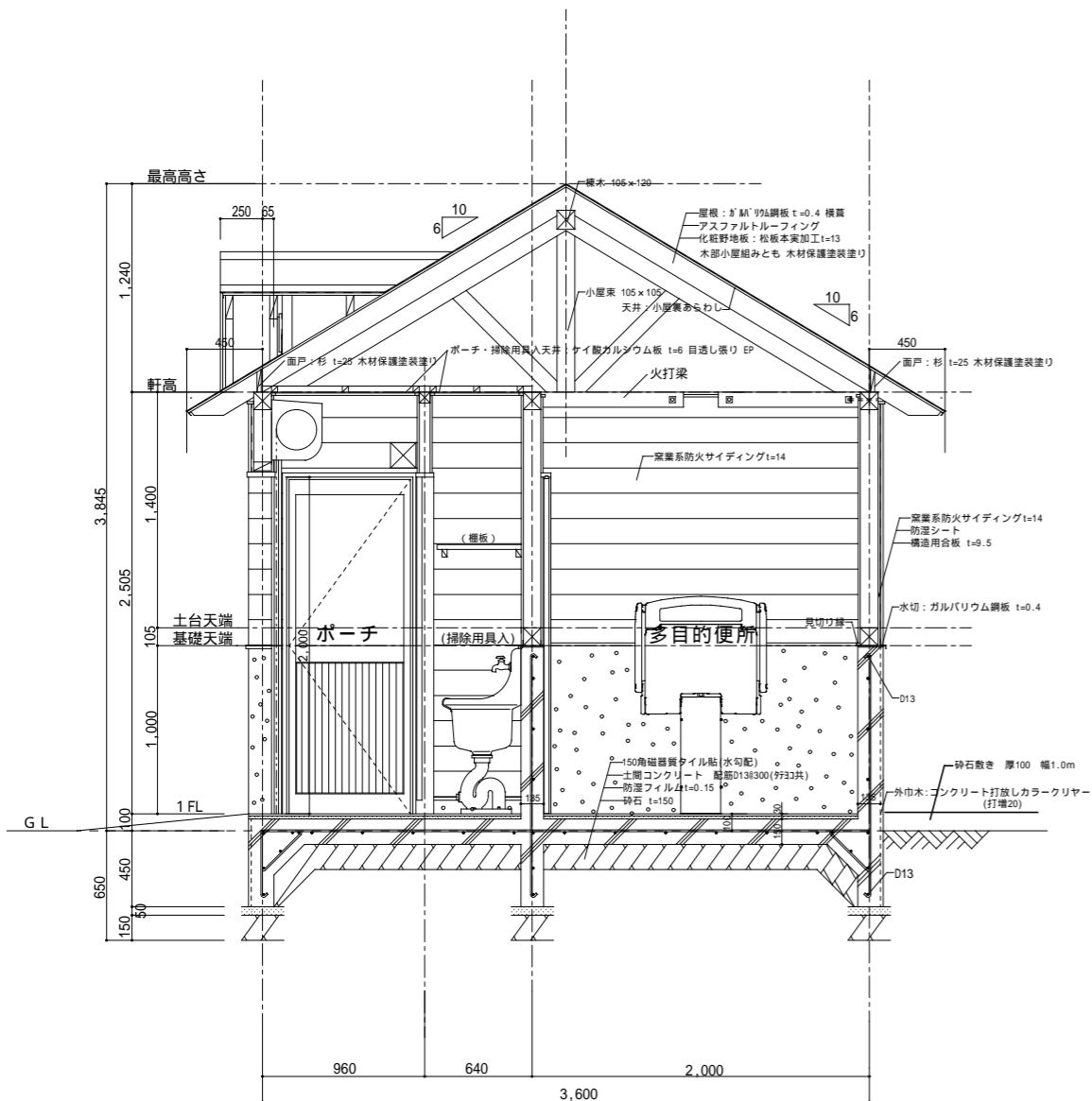
矩計図 SC/1:30
