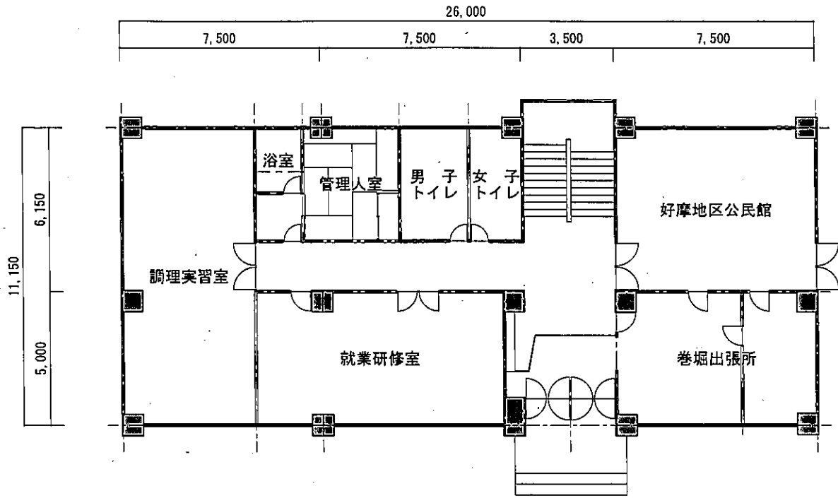
1階平面図 (改修前) 1:200
