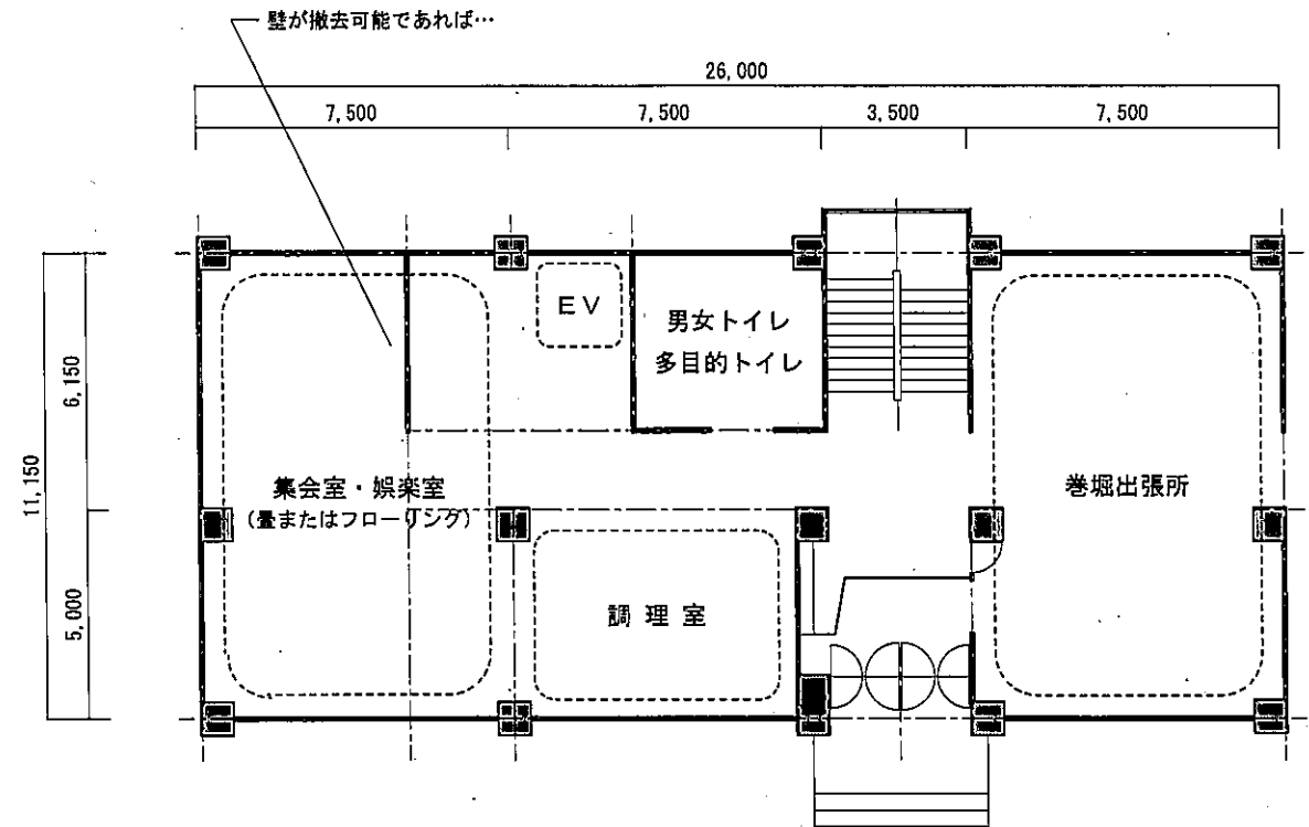
1階平面図 (改修後) 1:200
