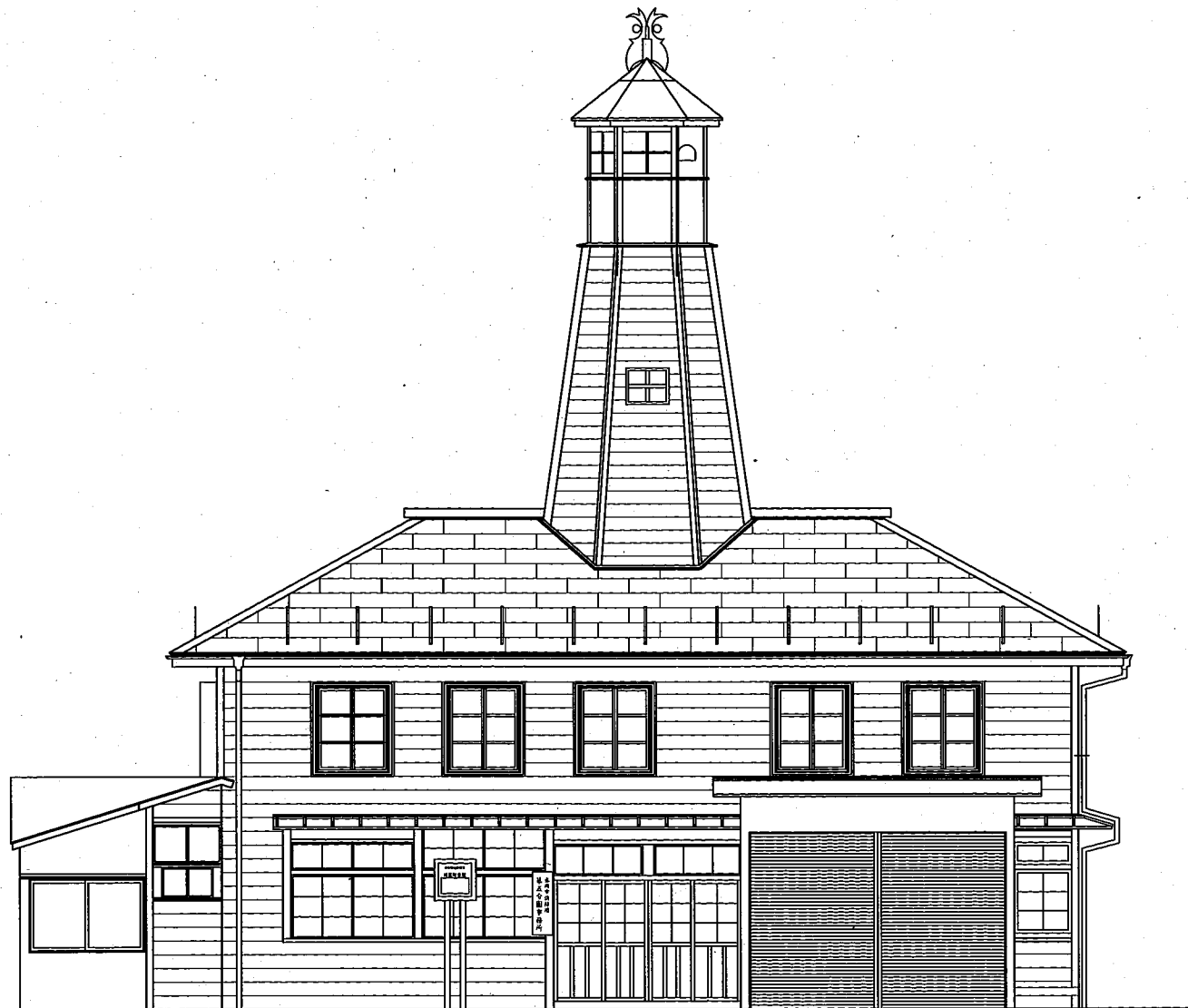
南立面图S=1/100
