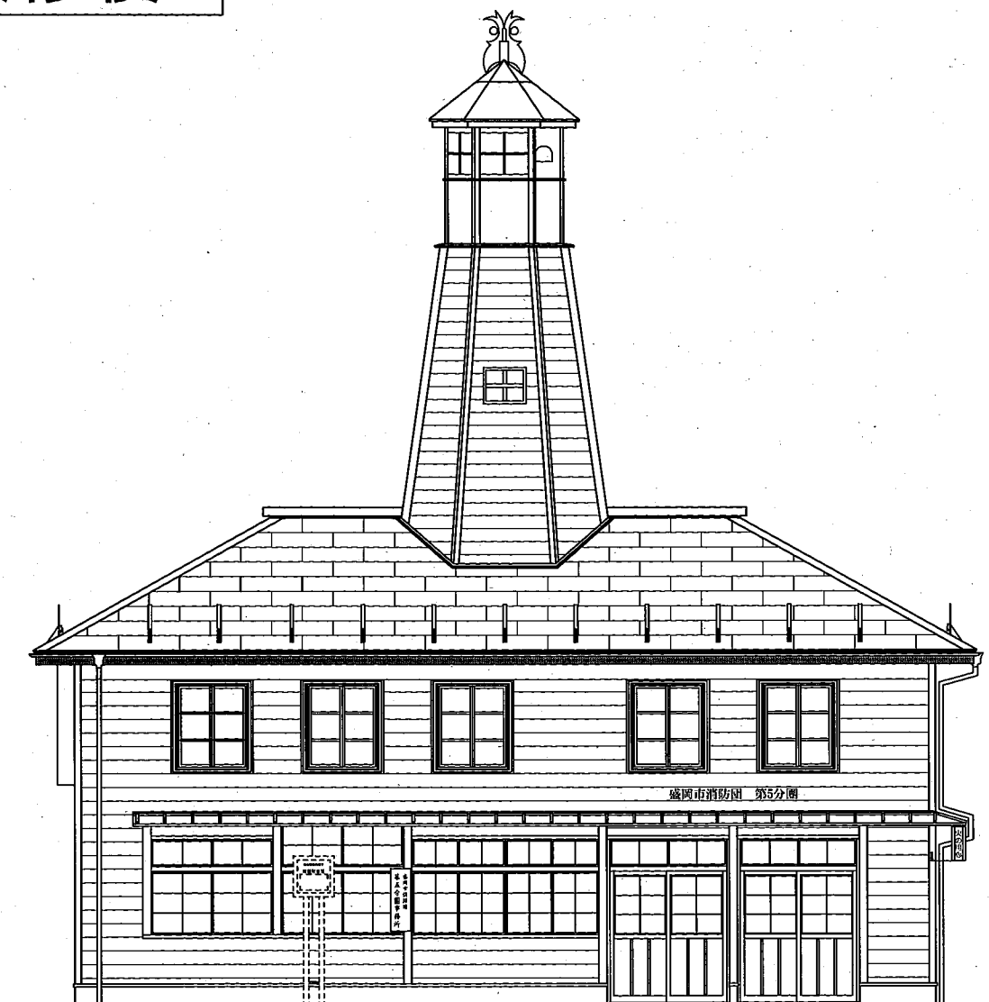
南立面図S=1/100
