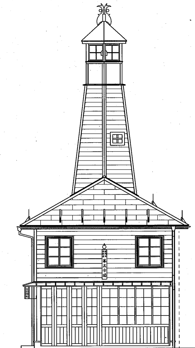
東立面図S=1/100
