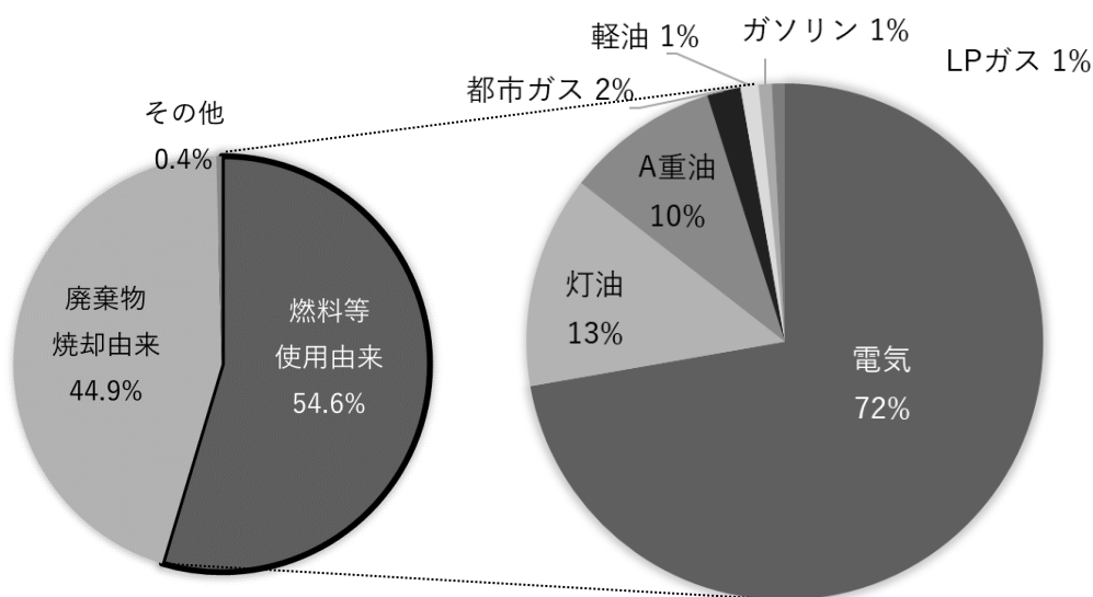
図4 温室効果ガス排出量の使用形態別内訳（令和元年度実績）
