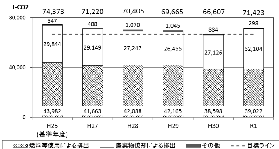
図3 平成27年度から令和元年度までの温室効果ガス排出量の推移
