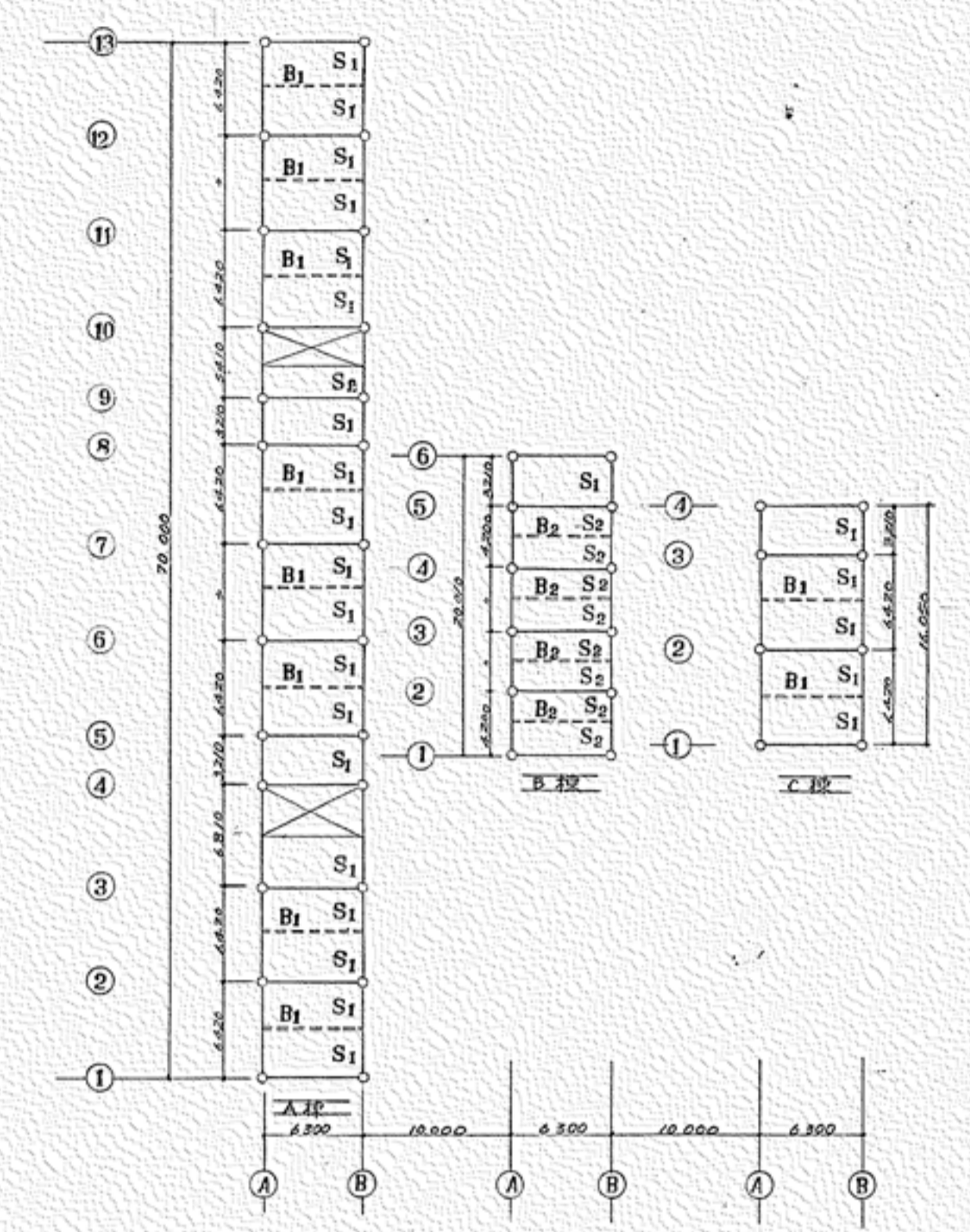
2階 小梁 スラブ KEY PLAN S 1:400
