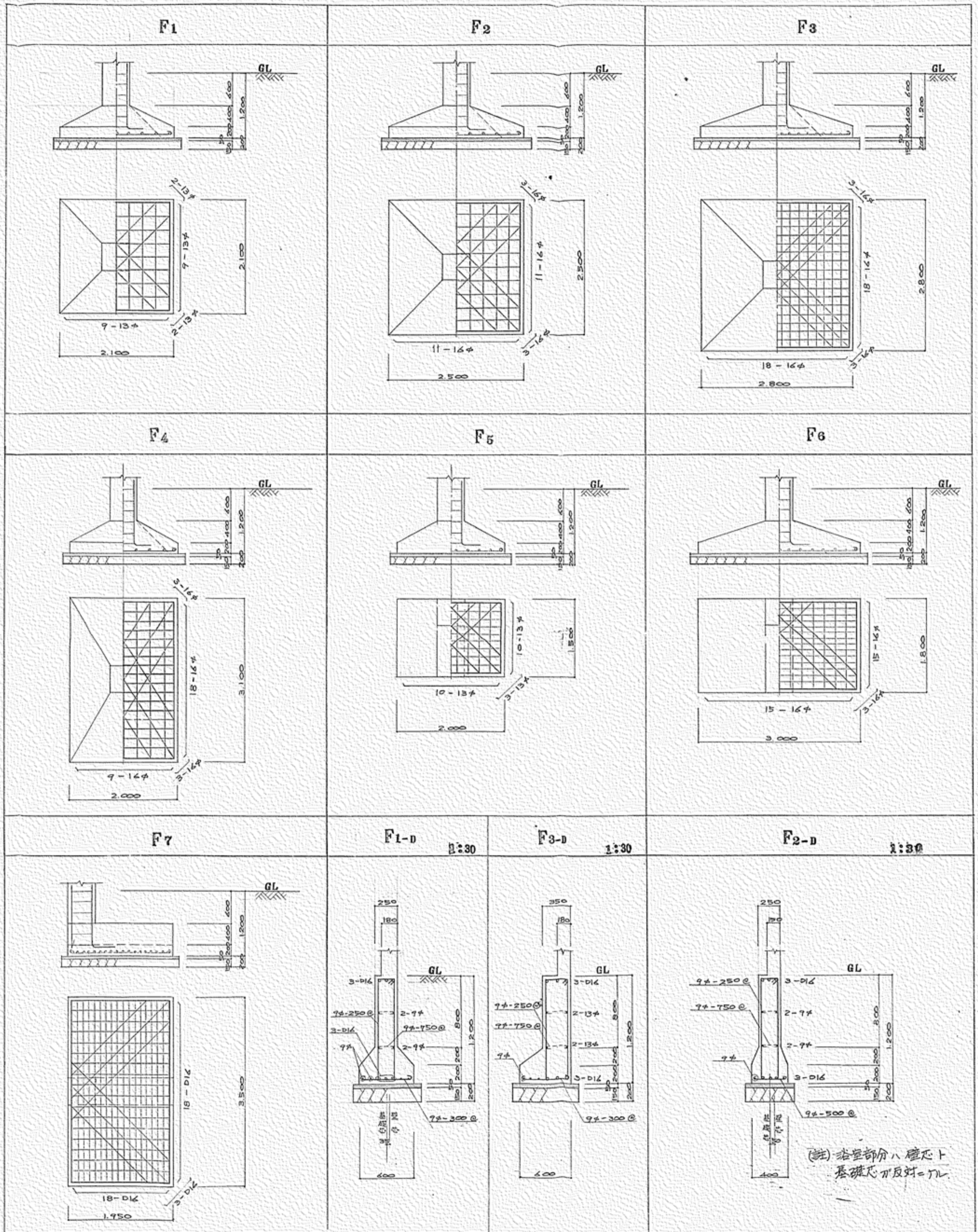
基礎リスト 1:50
