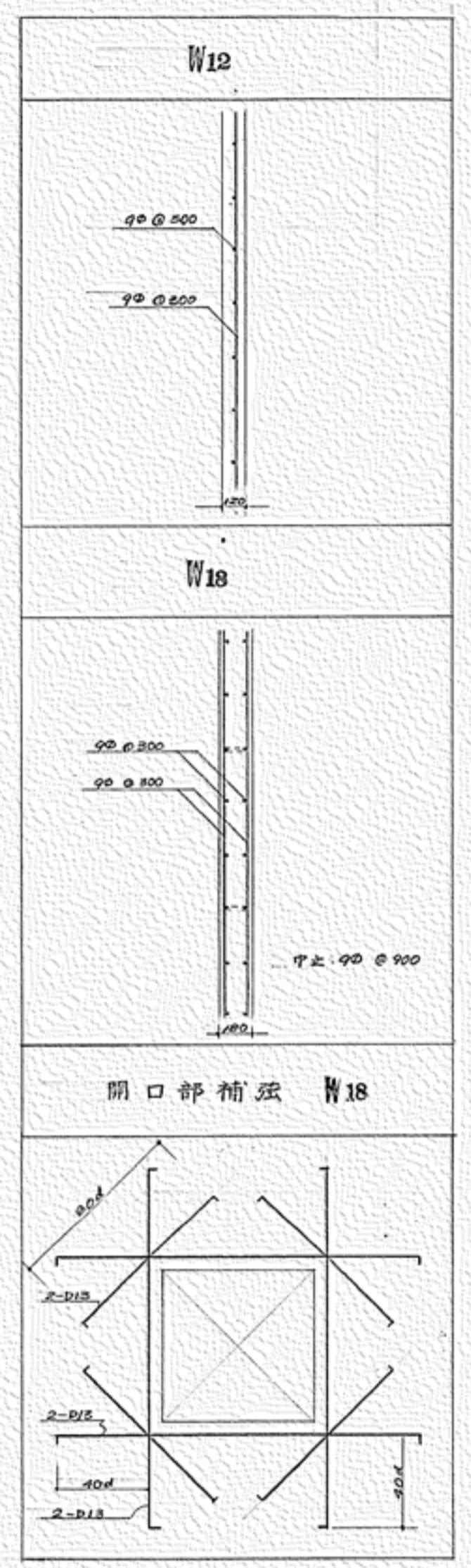
壁 リスト S 1:30
