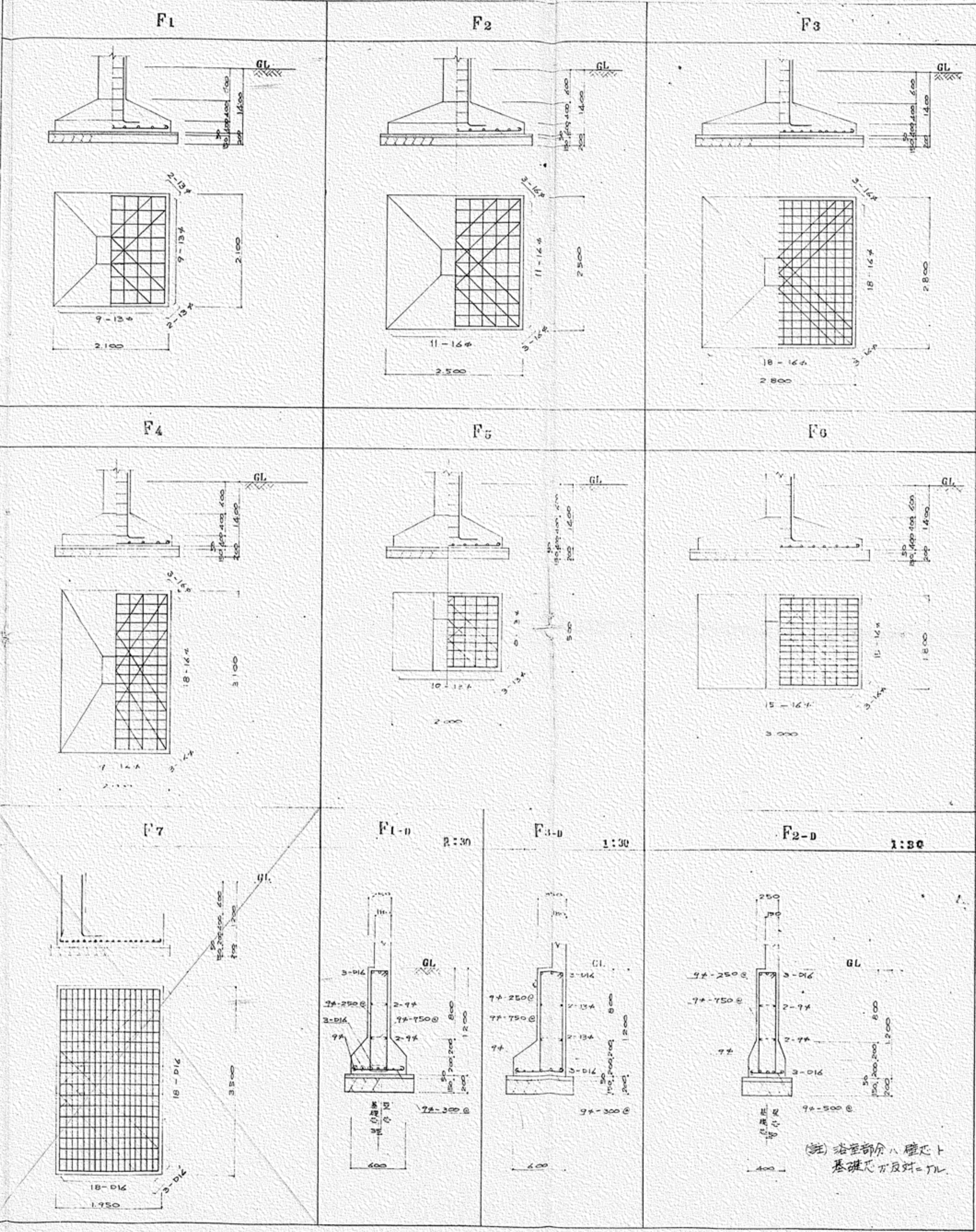
基礎リスト 1:50
