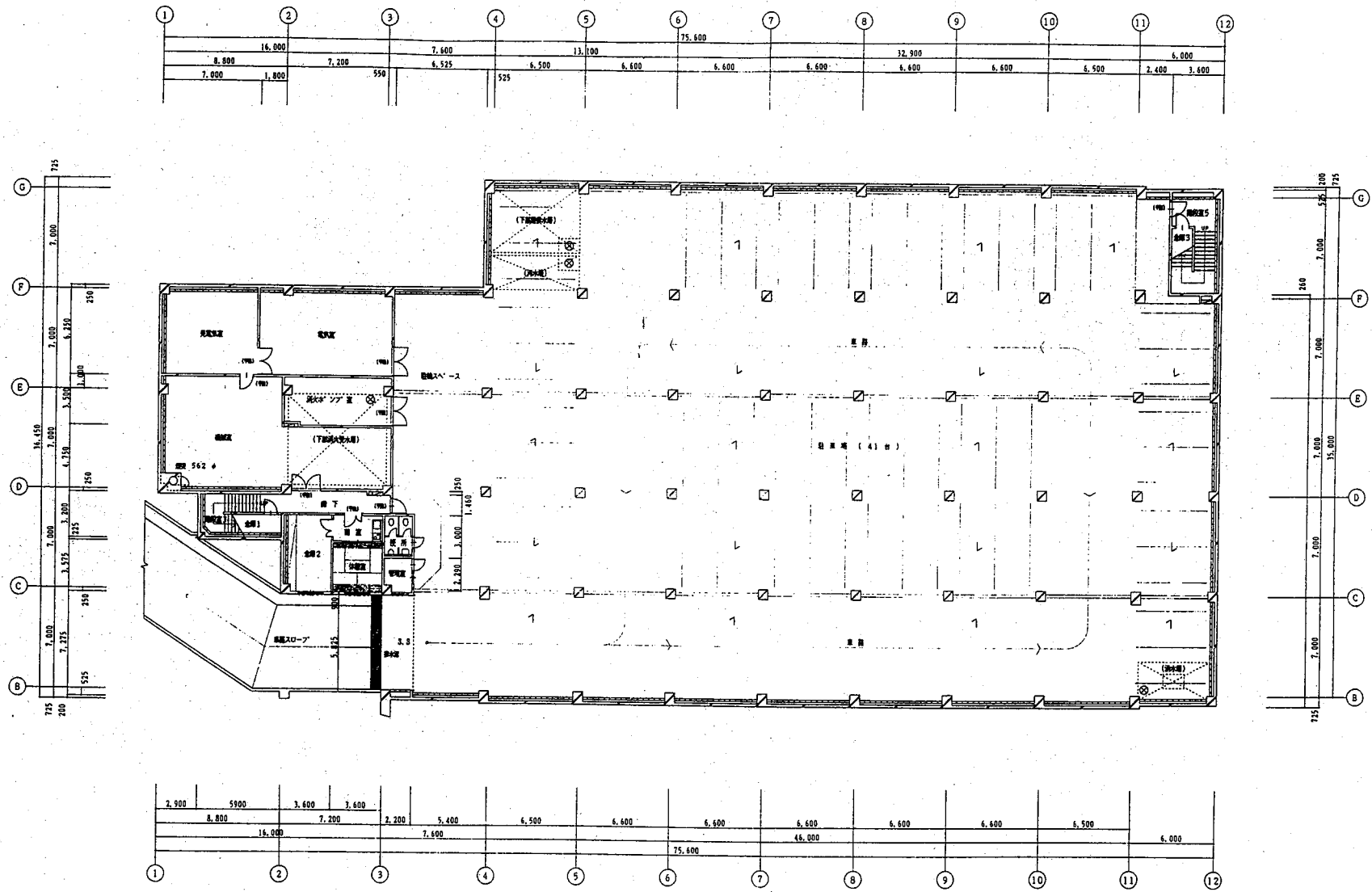
B 1 階平面図 1 : 150
