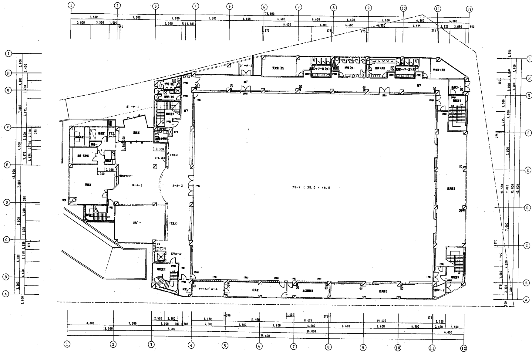
1階平面図 1:150
