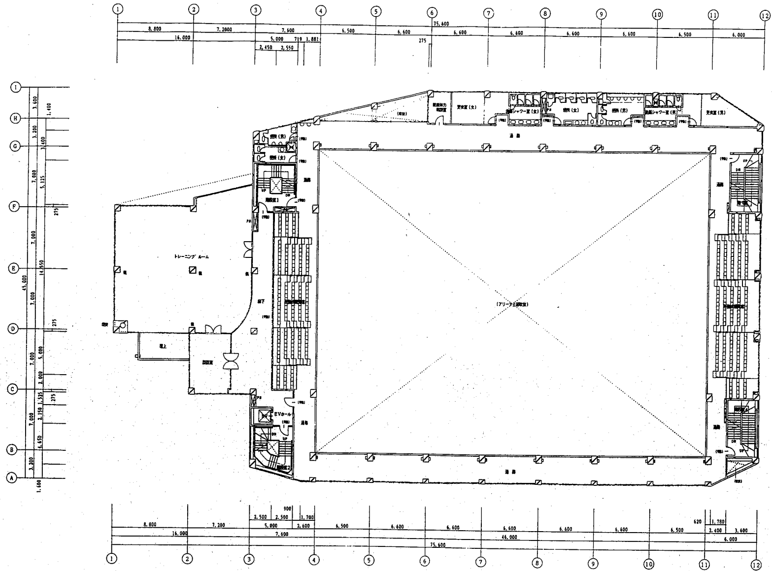
2階平面図 1:150
