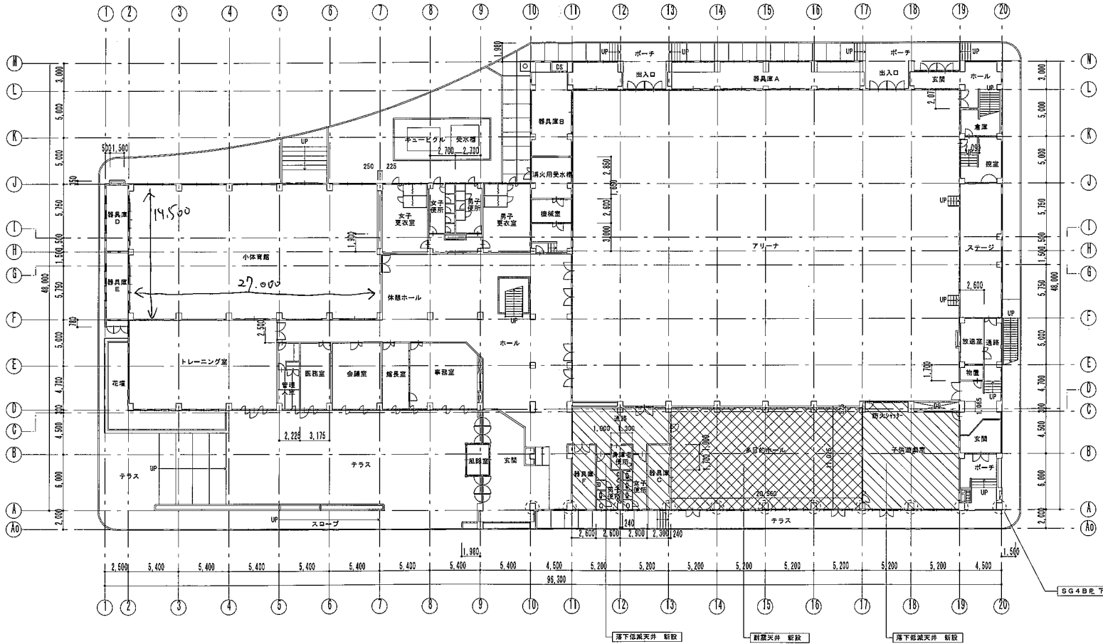
改修後 1階平面図 S=1:200
