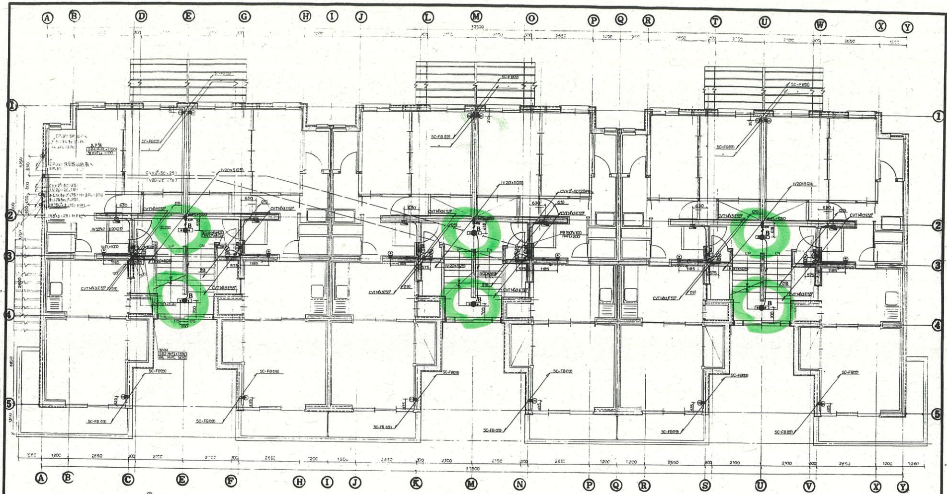
2階平面図 1:50
