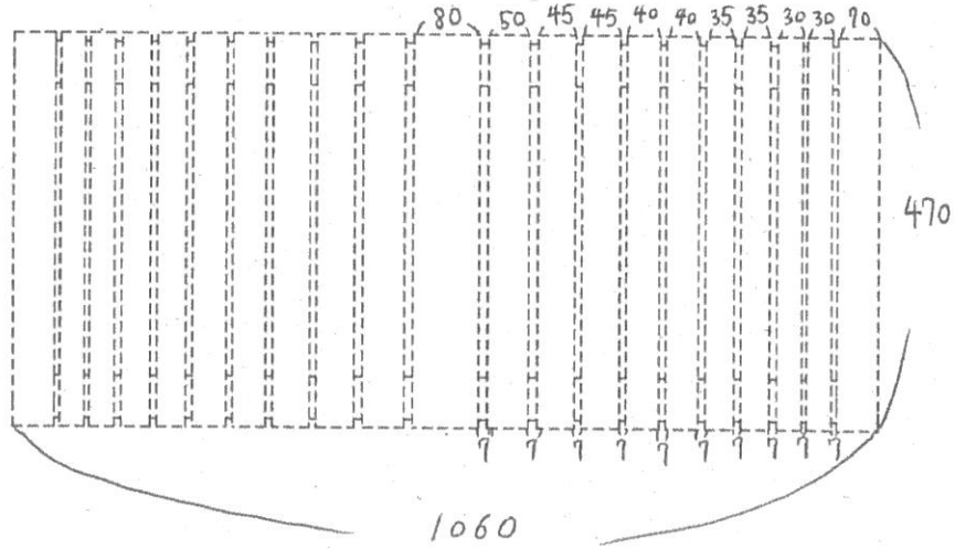
【正面図】
