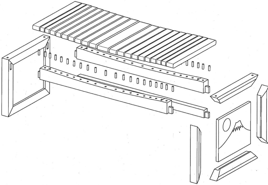
【参考分解斜視図】
