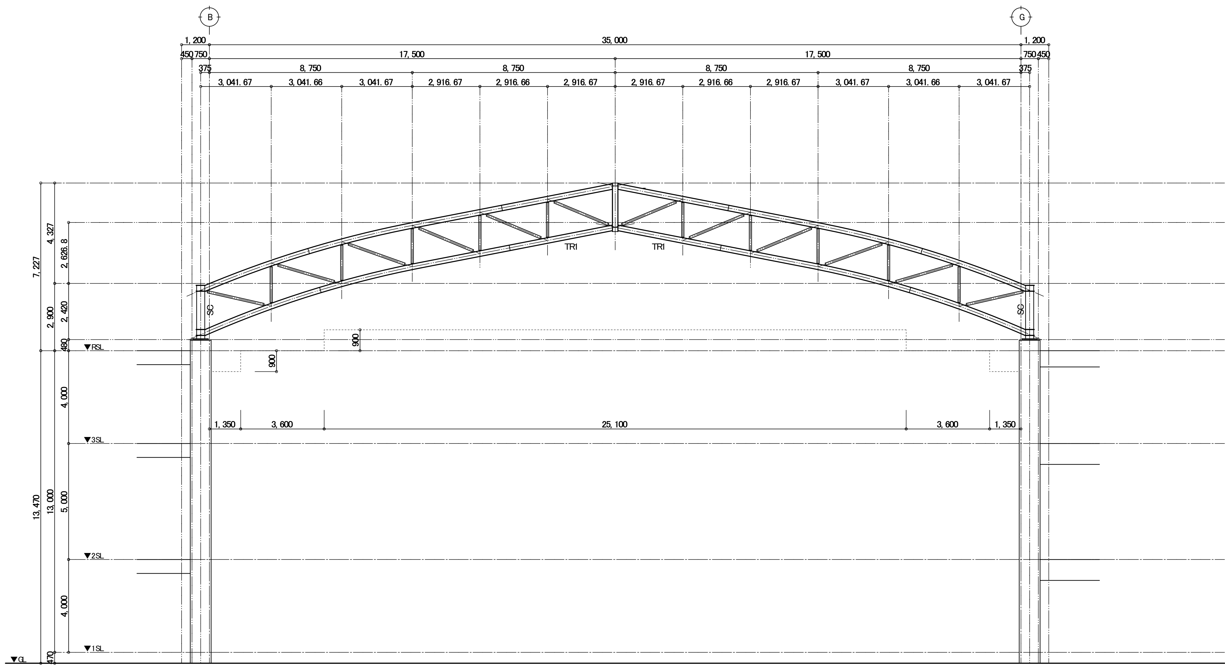
5・10通り 軸組図( 既存) 1: 100
