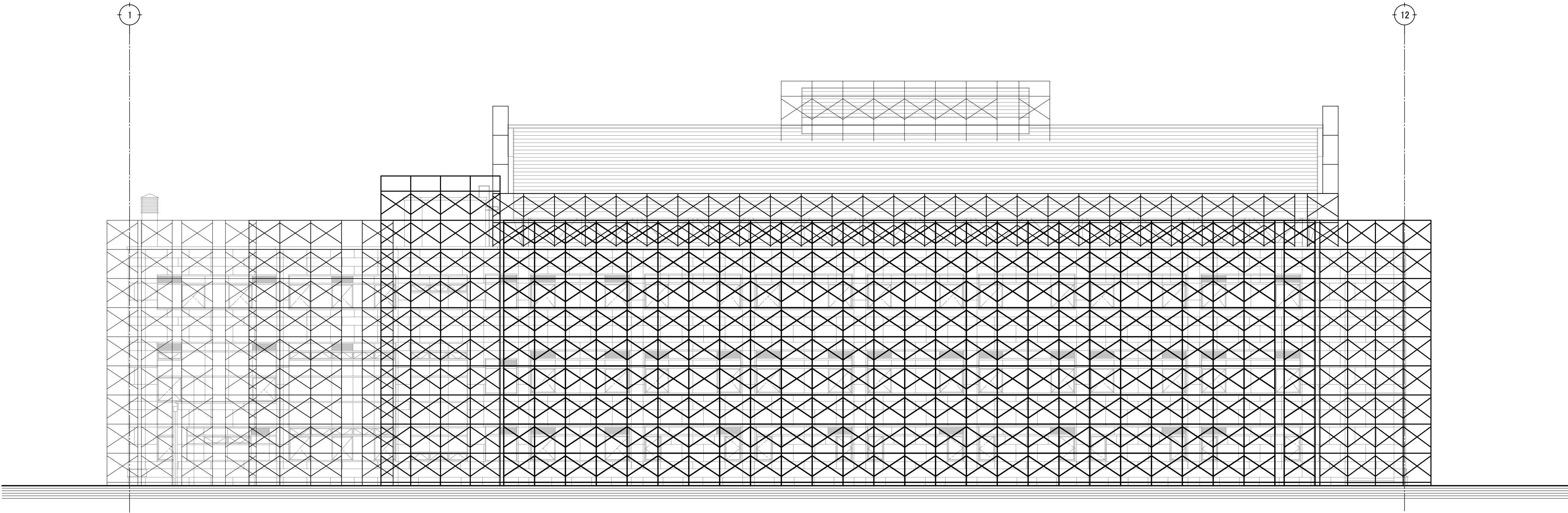
南側立面図 1: 150
