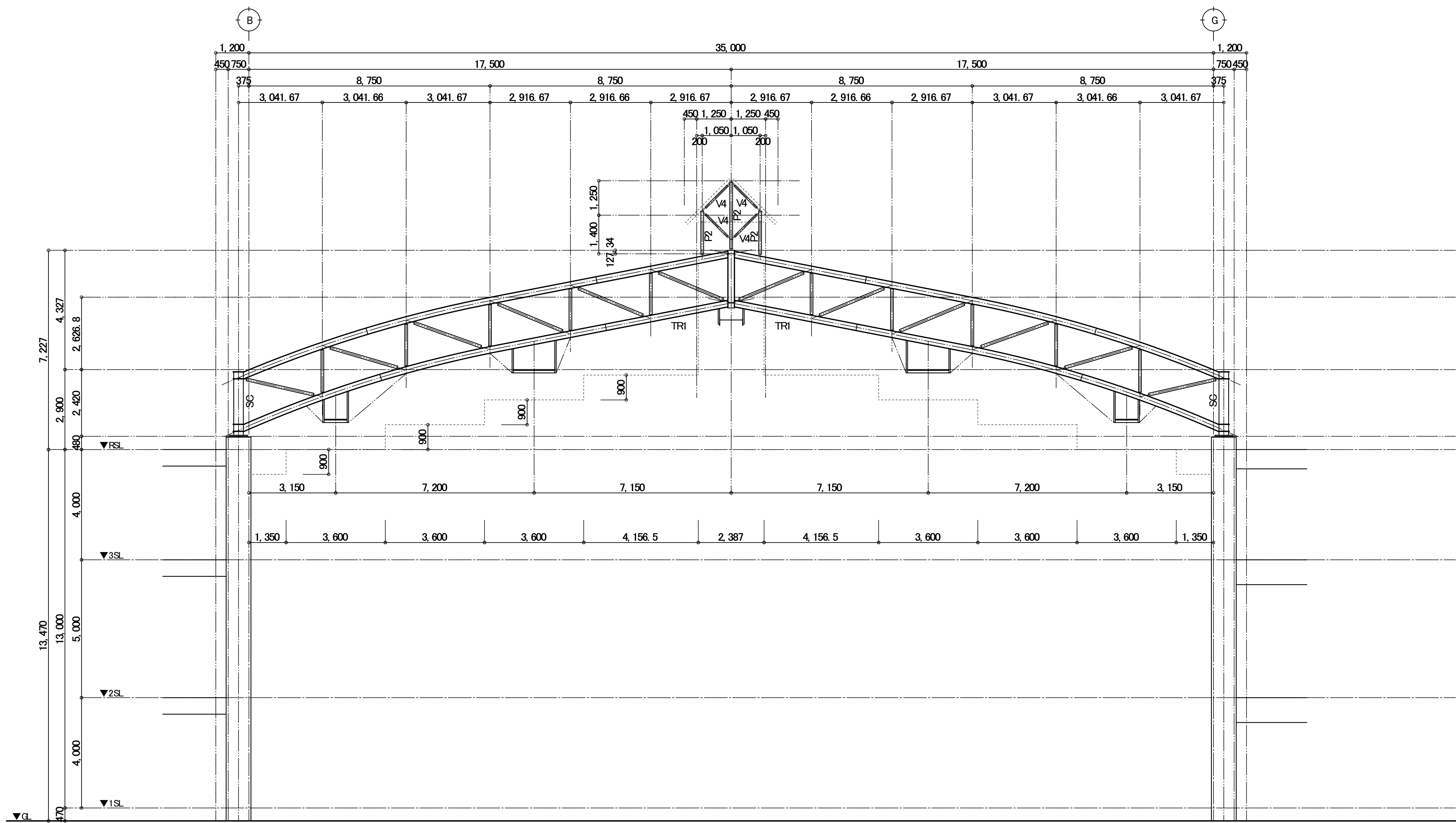
7・8通り 軸組図(既存) 1:100
