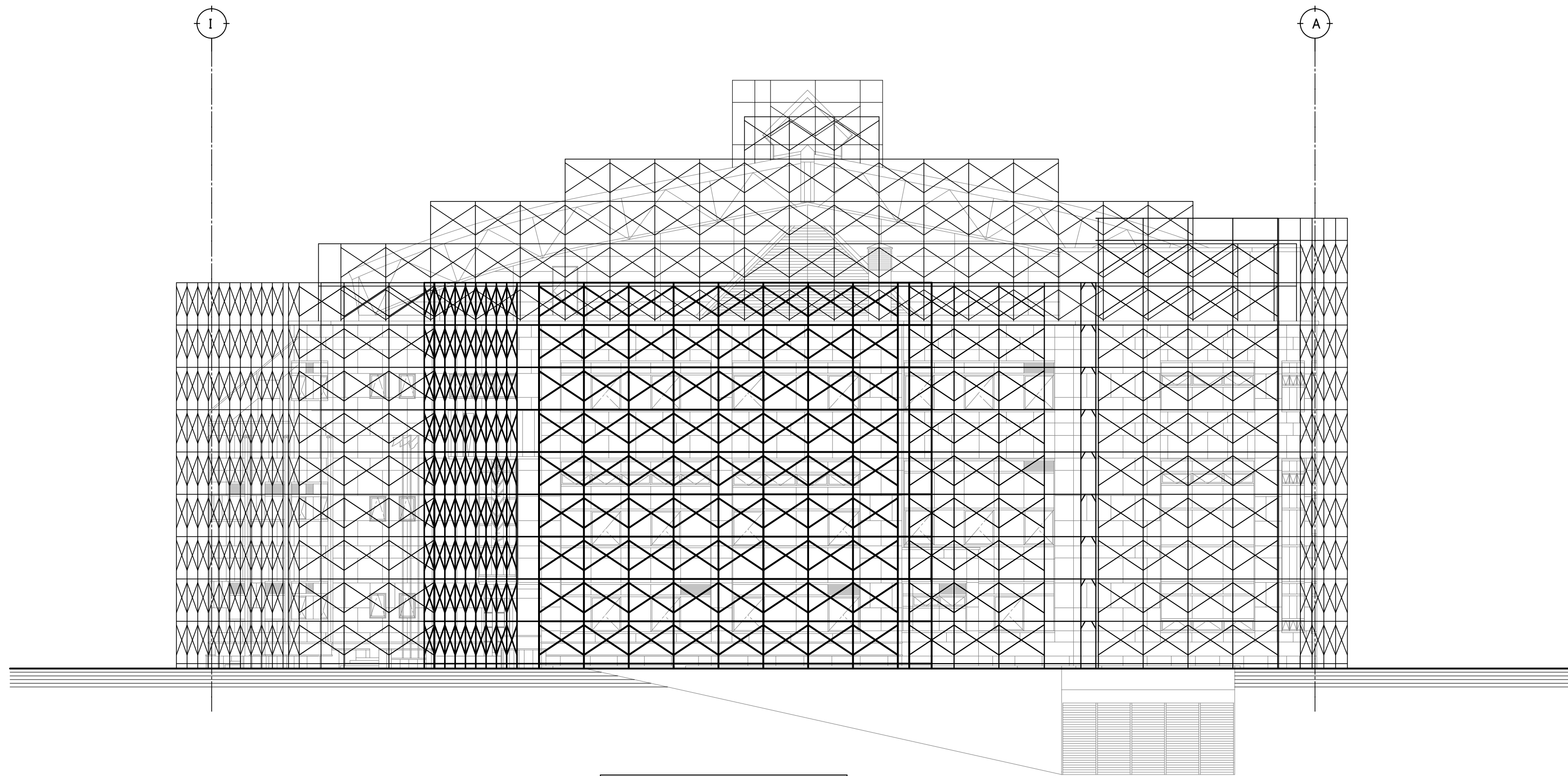
西側立面図 1: 150
