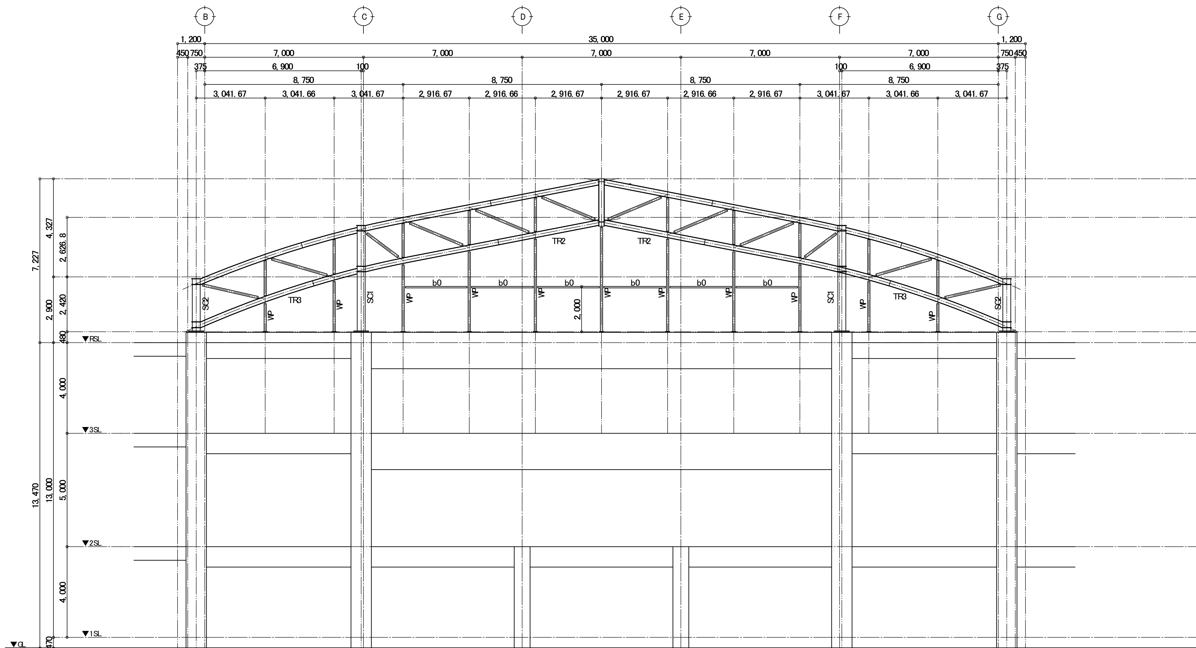
4・11通り 軸組図(既存) 1:100
