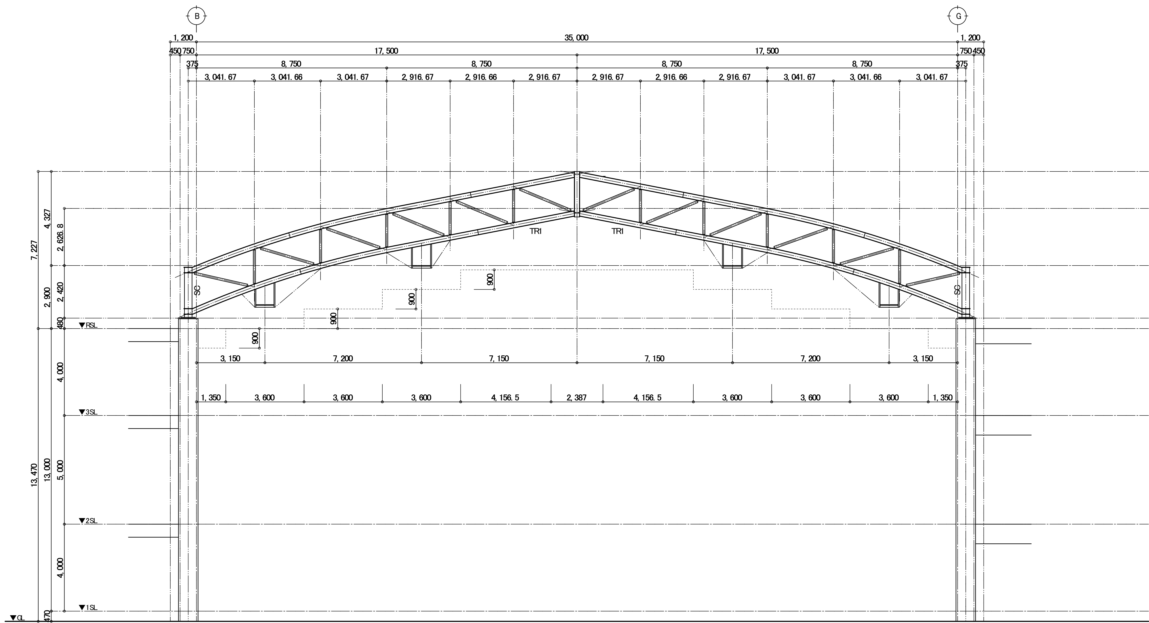
6・9通り 軸組図(既存) 1:100
