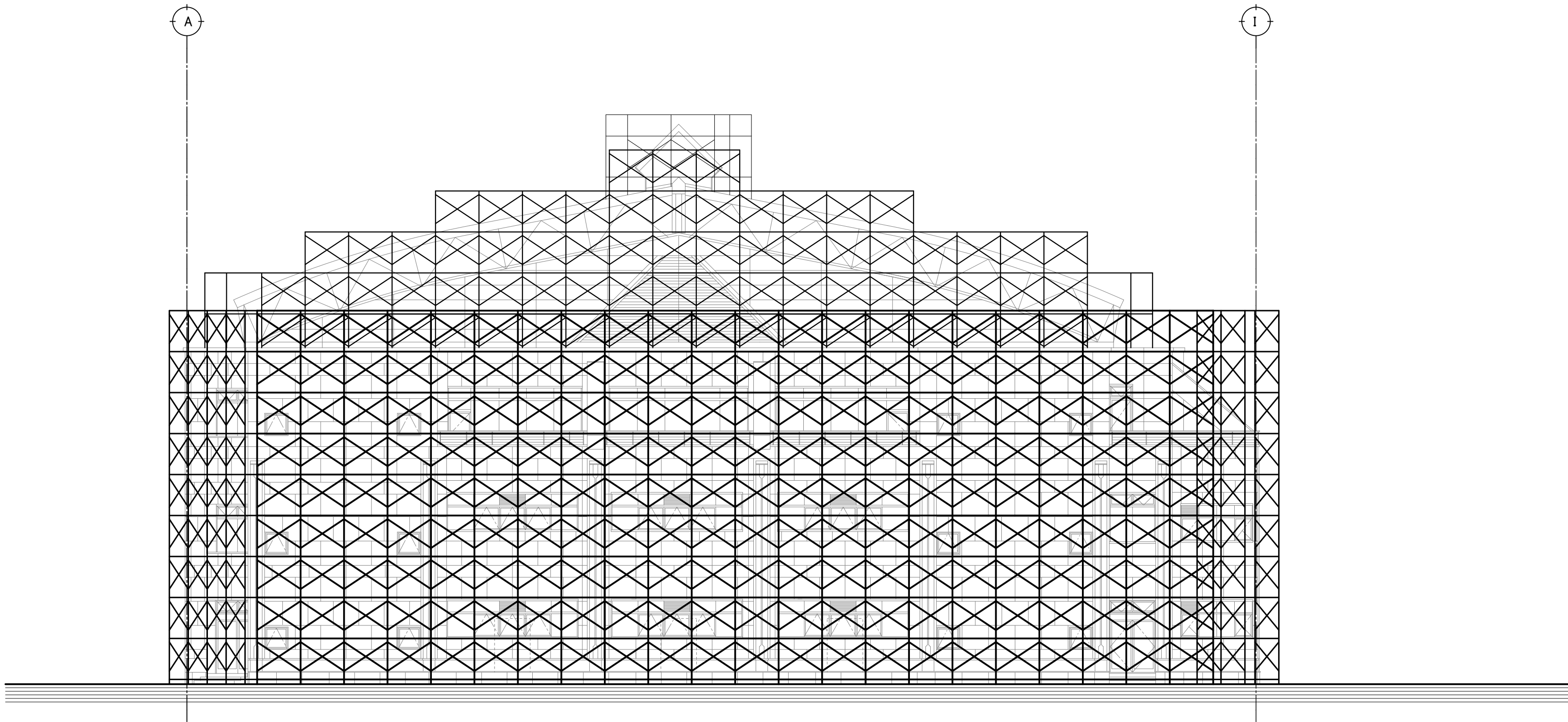
東側立面図 1: 150
