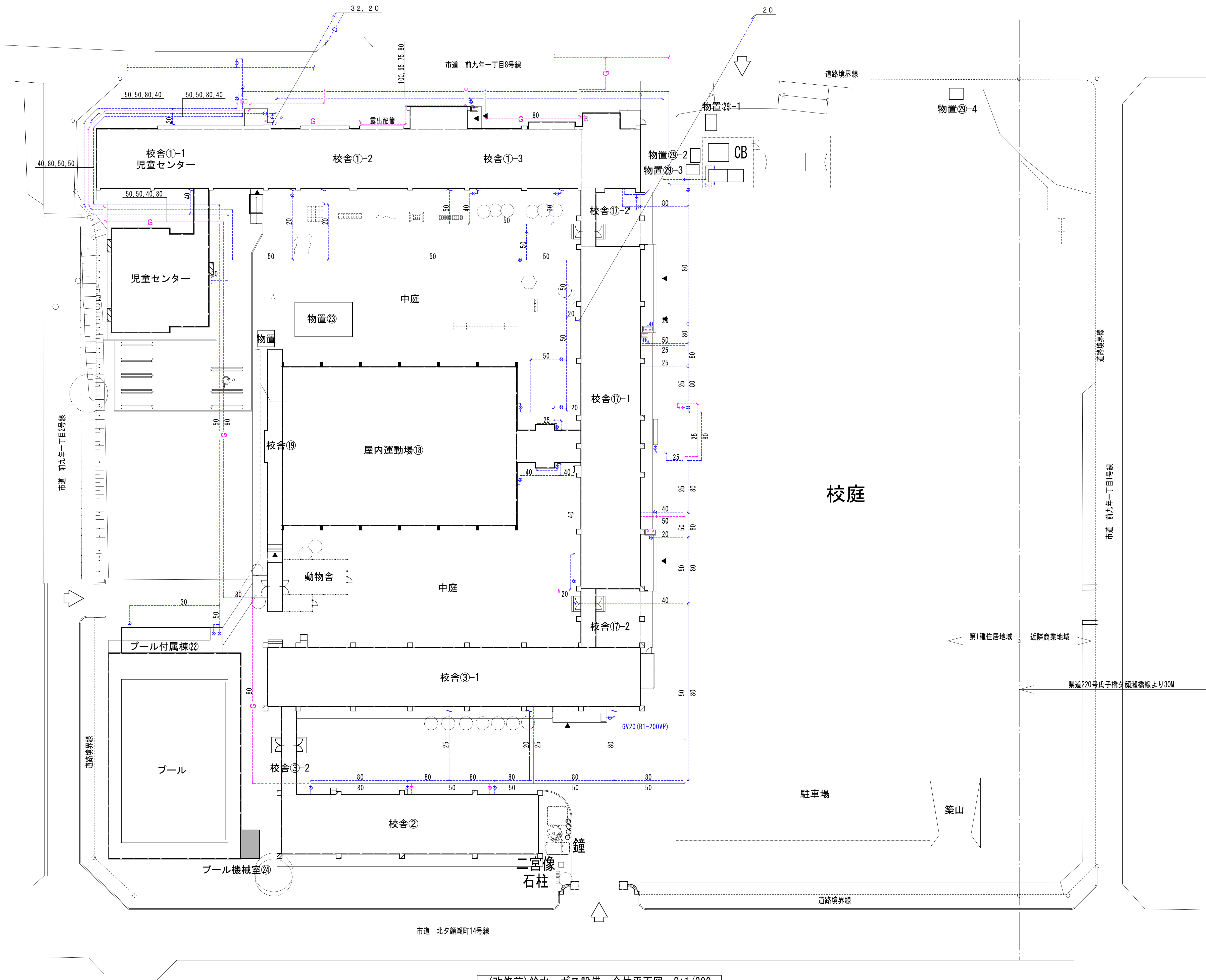
(改修前)給水・ガス設備 全体平面図 S:1/300
