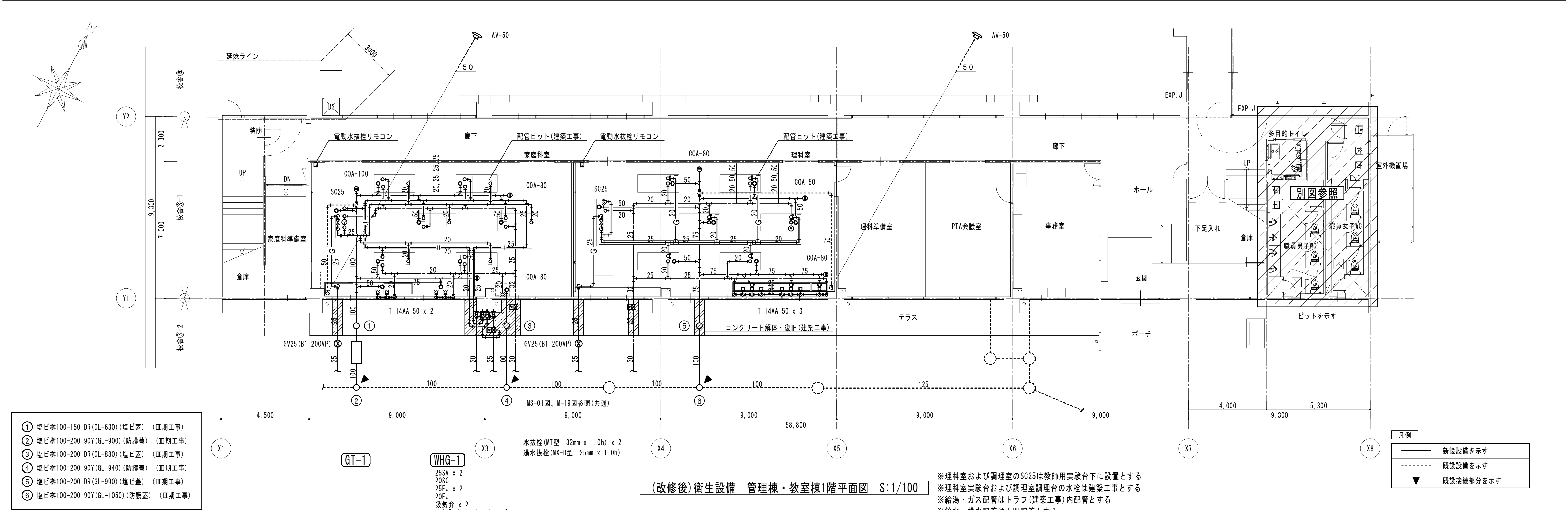
(改修前)衛生設備 管理棟・教室棟1階平面図 S:1/100
