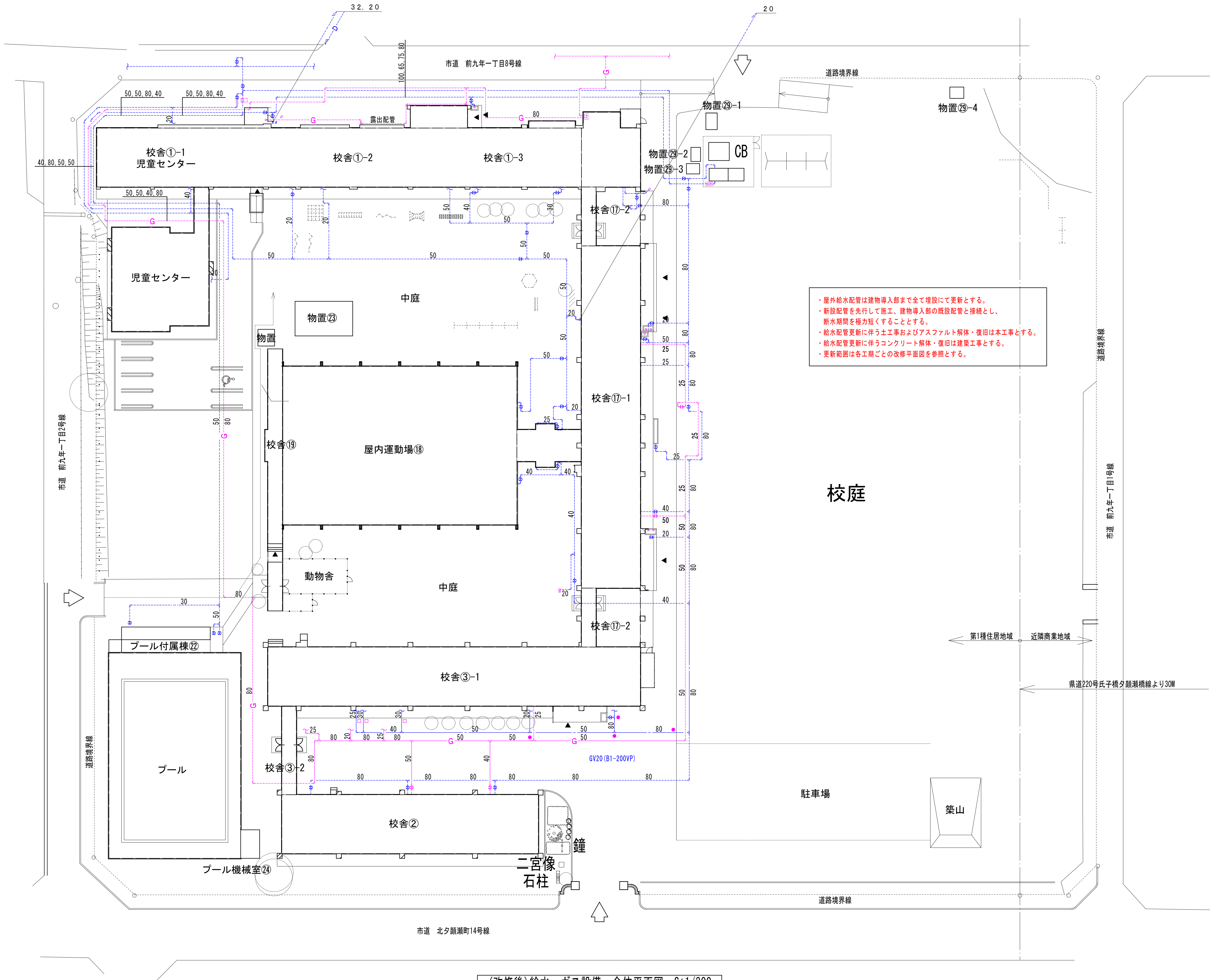
(改修後)給水・ガス設備 全体平面図 S:1/300
