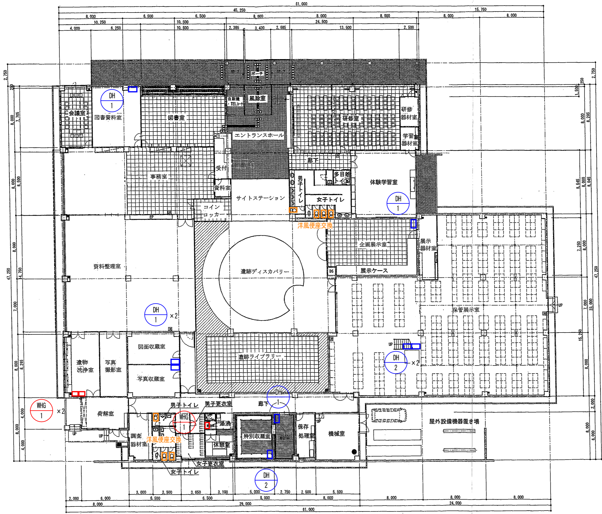
1階平面図
