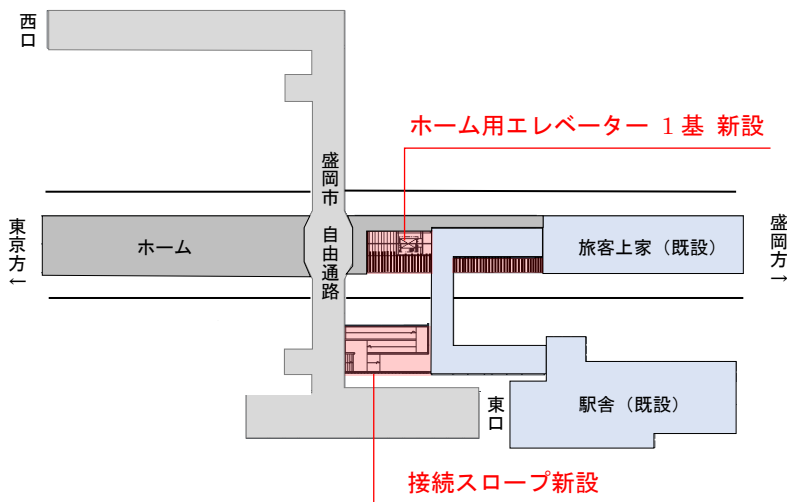
【平面計画】
