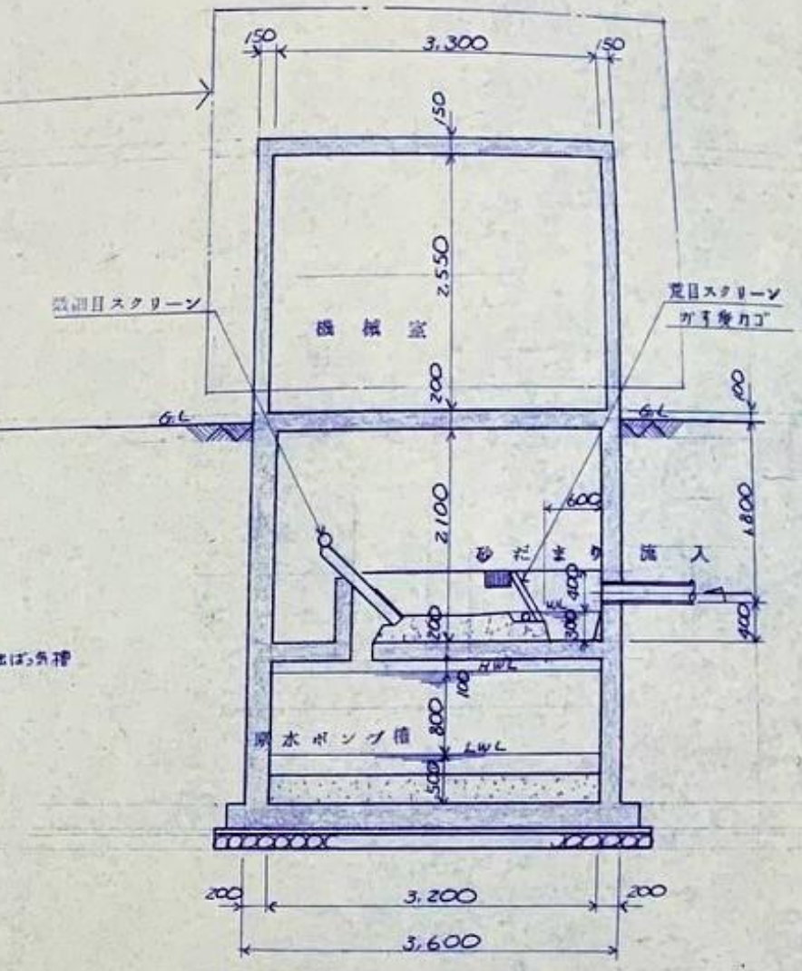
B-B断面図 1:50
