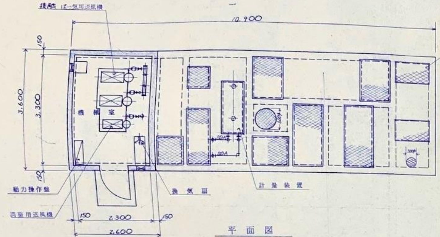
平面図 1:50
