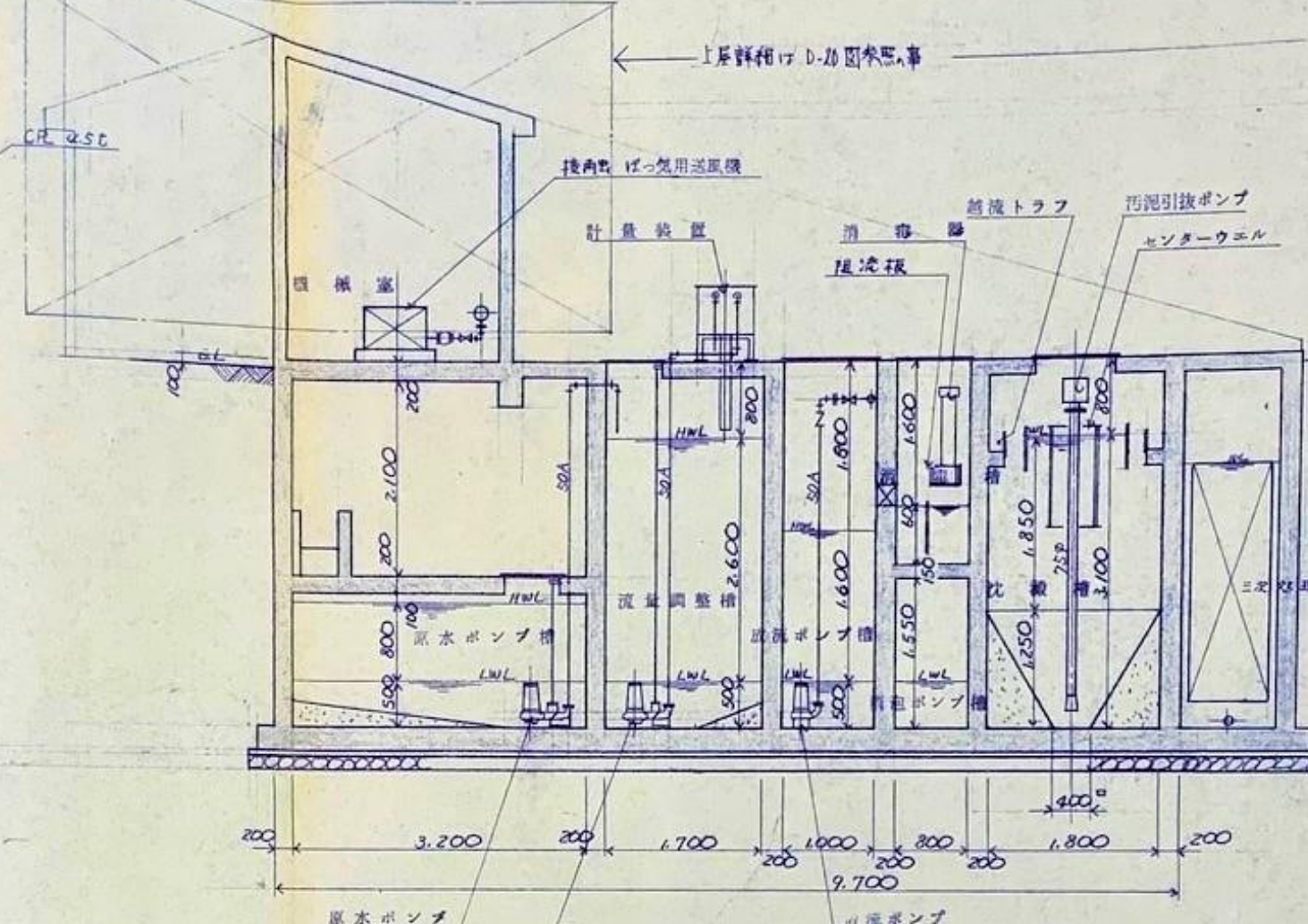
A-A断面図 1:50
