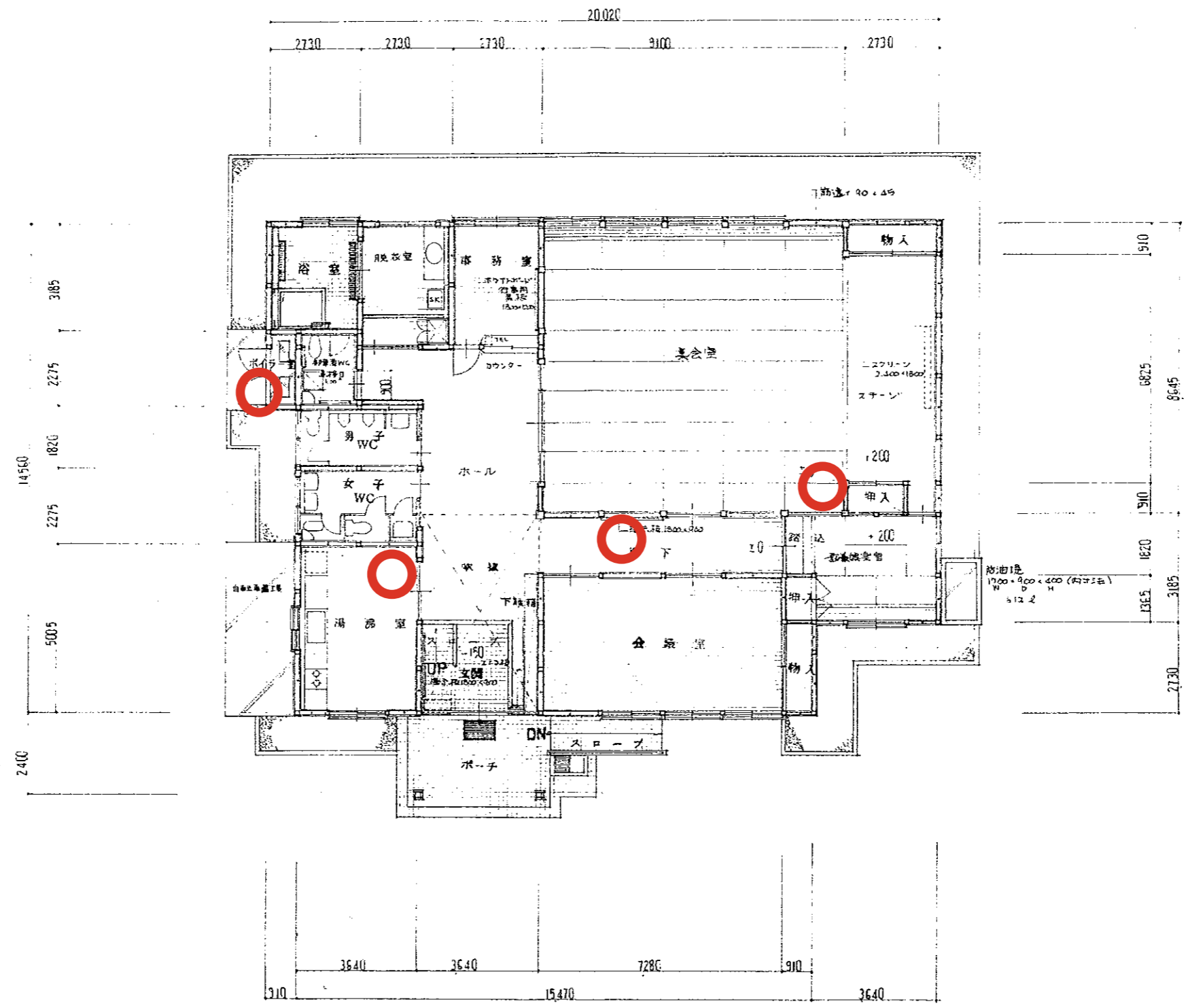
平面図 1:100
