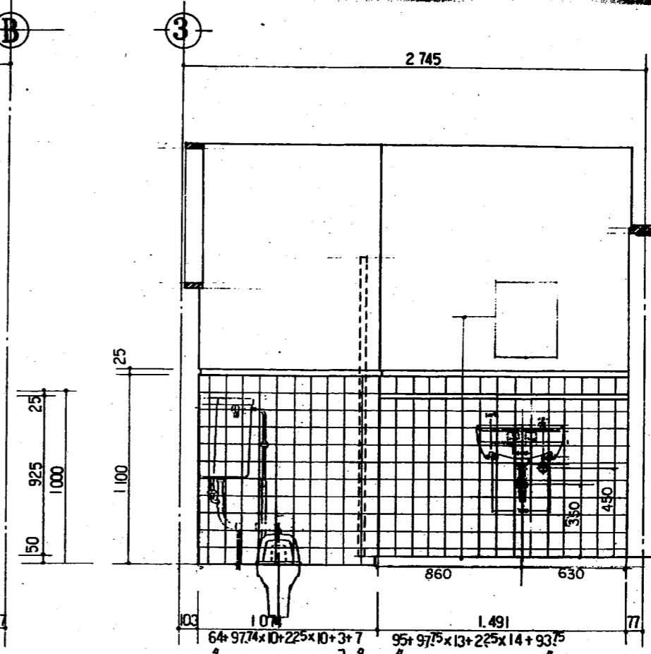
C面 展開図
