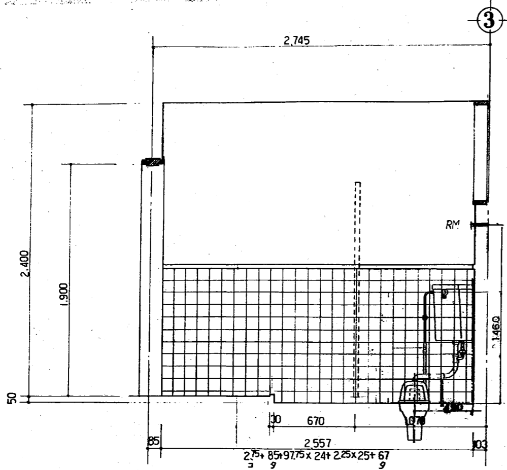
A面 展開図
