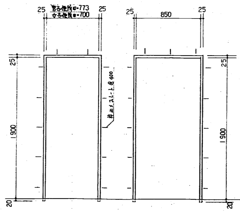
便所 ドア仕様図 1:20
