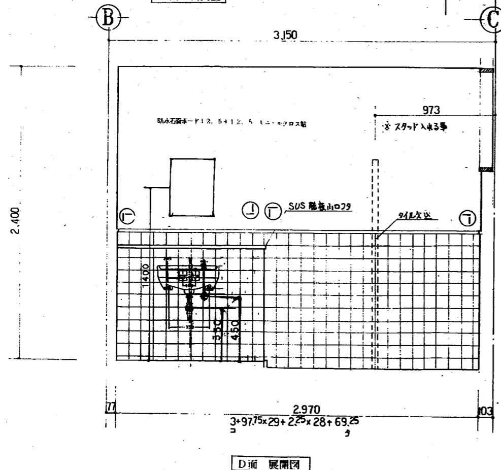
1階女子便所 展開図 1:5
