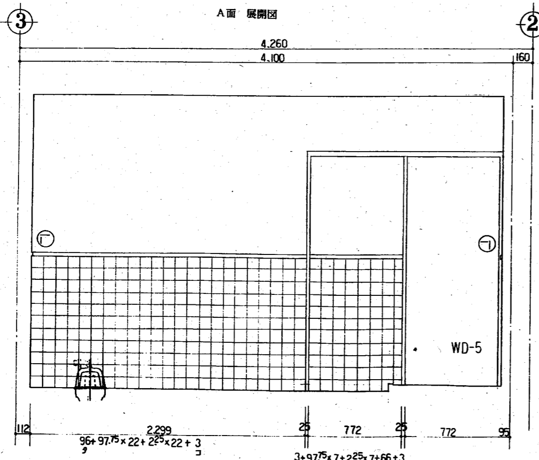
C面 展開図
