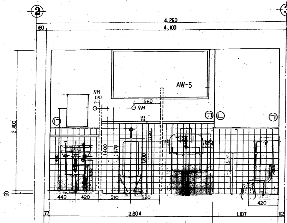
A面 展開図
