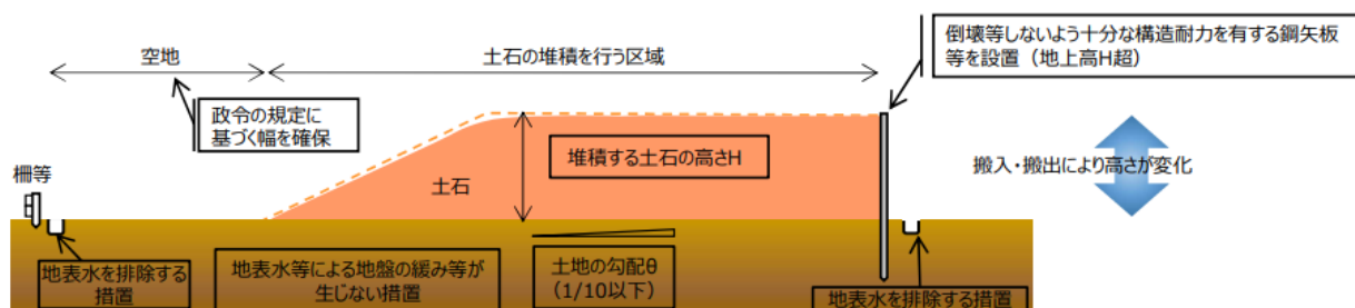
図9-3 鋼矢板等の設置の例 (出典：国土交通省 HP)
