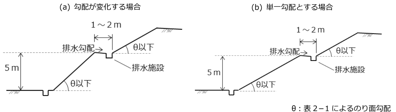
図2-6 切土のり面の形状
