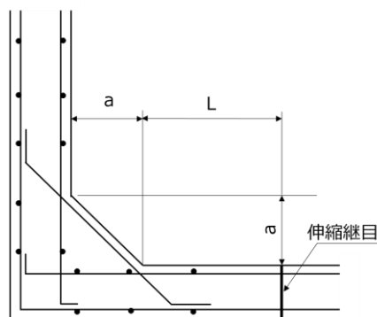
図 4-4 伸縮継目及び隅角部の補強
