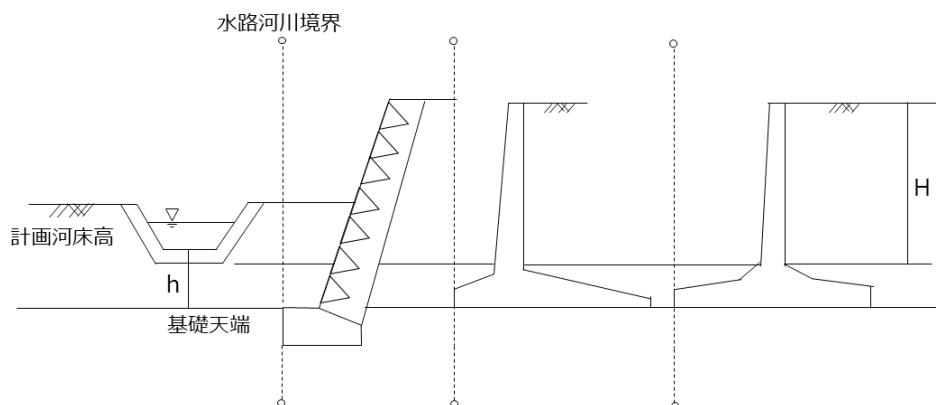
図 4-3 水路等に近接して擁壁を設置する場合の根入れ
