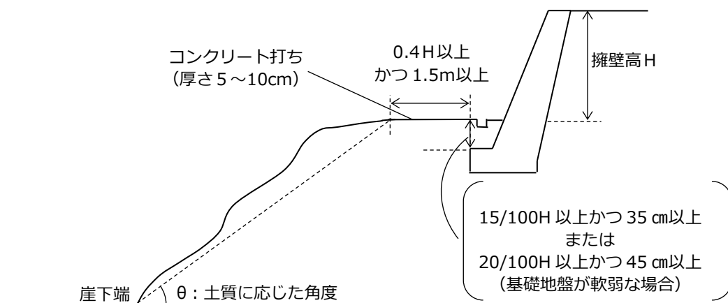
図 3-2 斜面上部に設置する擁壁
