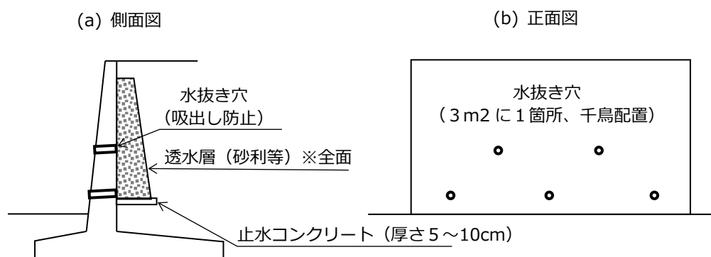
図 4-6 コンクリート造の擁壁における水抜き穴及び透水層の配置
