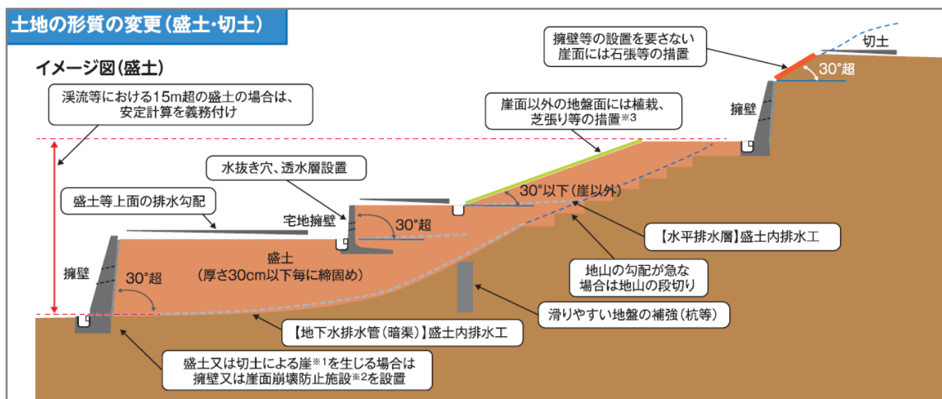
図 1 - 1 宅地造成、特定盛土等に関する工事の技術的基準（出典：盛土規制法パンフレット（国））
