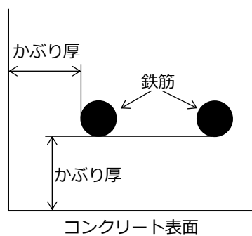
図 4 - 5 鉄筋のかぶり厚さ
