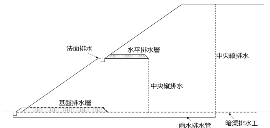
図 8－1 盛土の排水施設の概要
