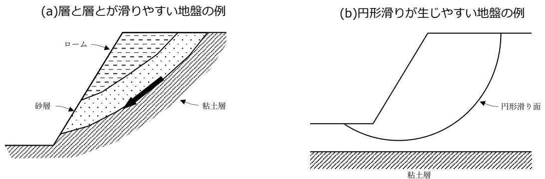
図2－8 滑りやすい切土地盤の例
