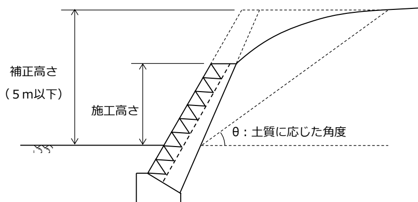
図 5 - 2 上部に斜面がある場合の練積み造擁壁
