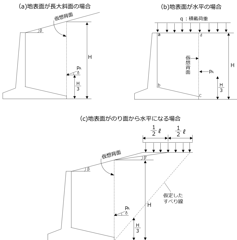
図 4 - 1 土圧作用位置の例
