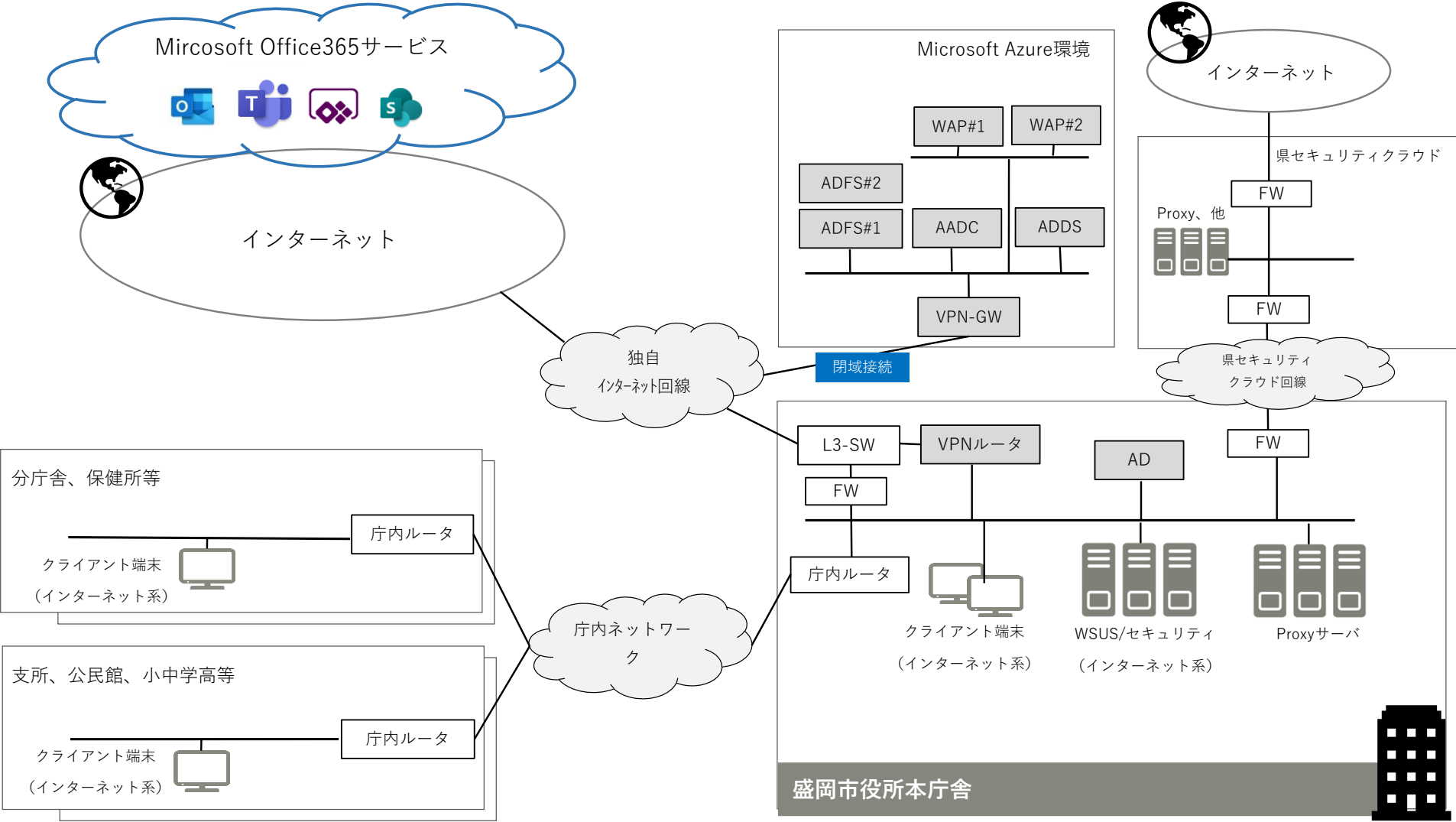
別紙3 既存システム構成図
