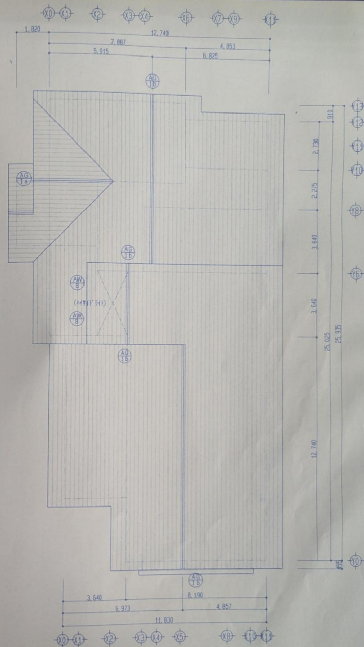
建具・家具配置図 1/100
