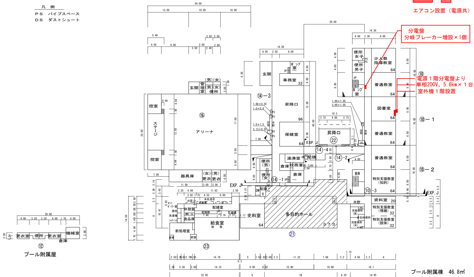
1階平面図
