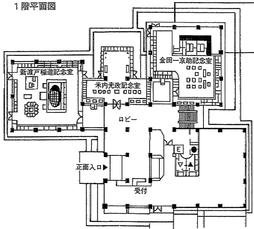
2 階平面図
