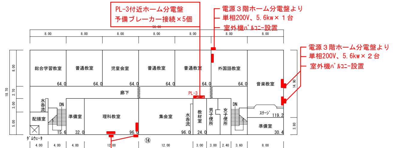
2 階 平 面 図
