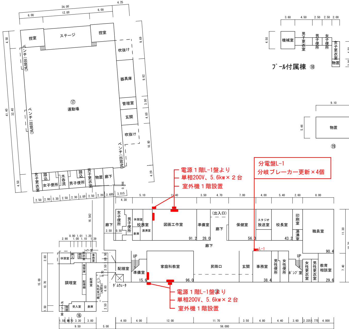
1 階 平 面 図
