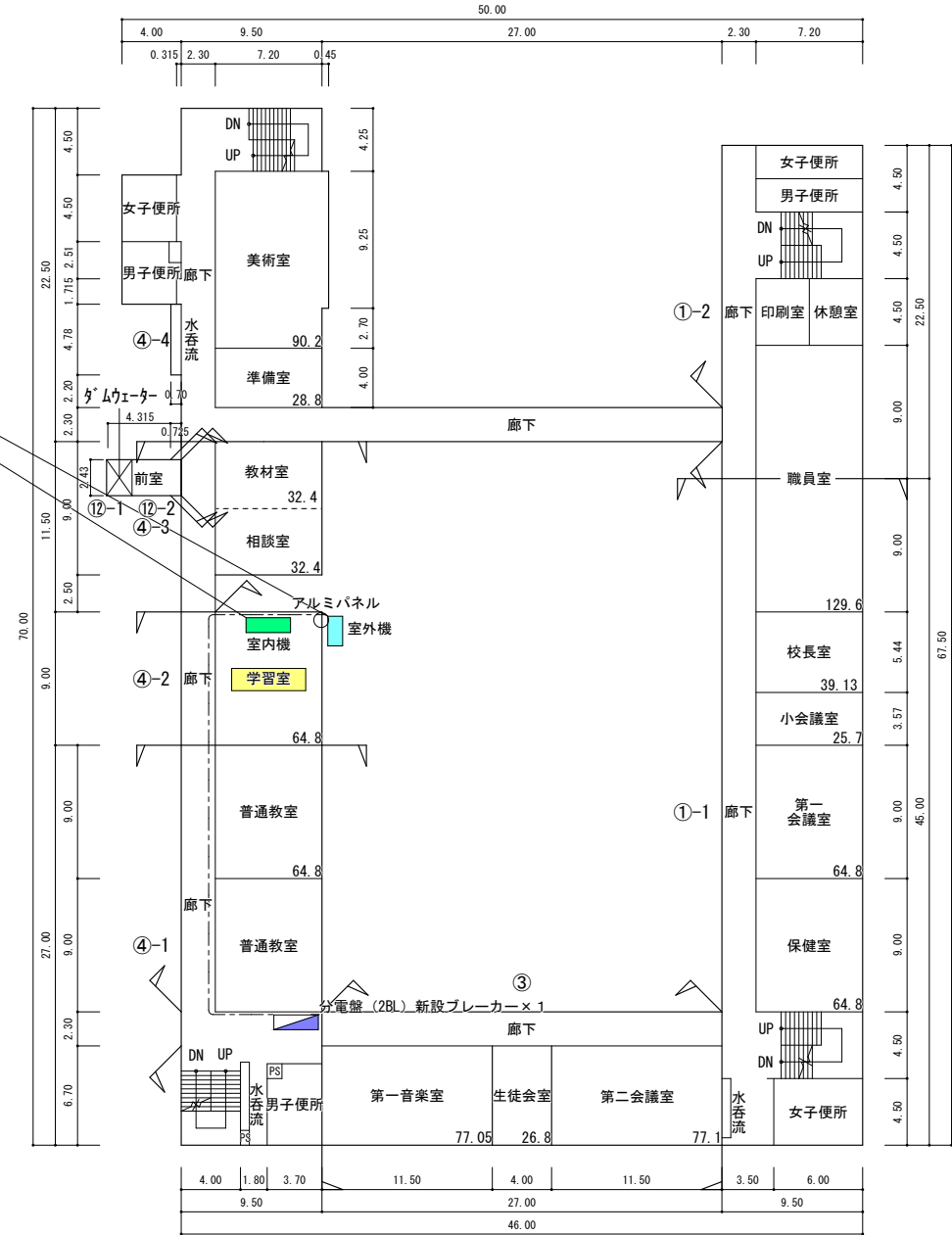
2 階 平 面 図
