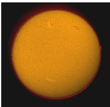
写真左：H \alpha 光による太陽全景 写真右：白色光による太陽全景
